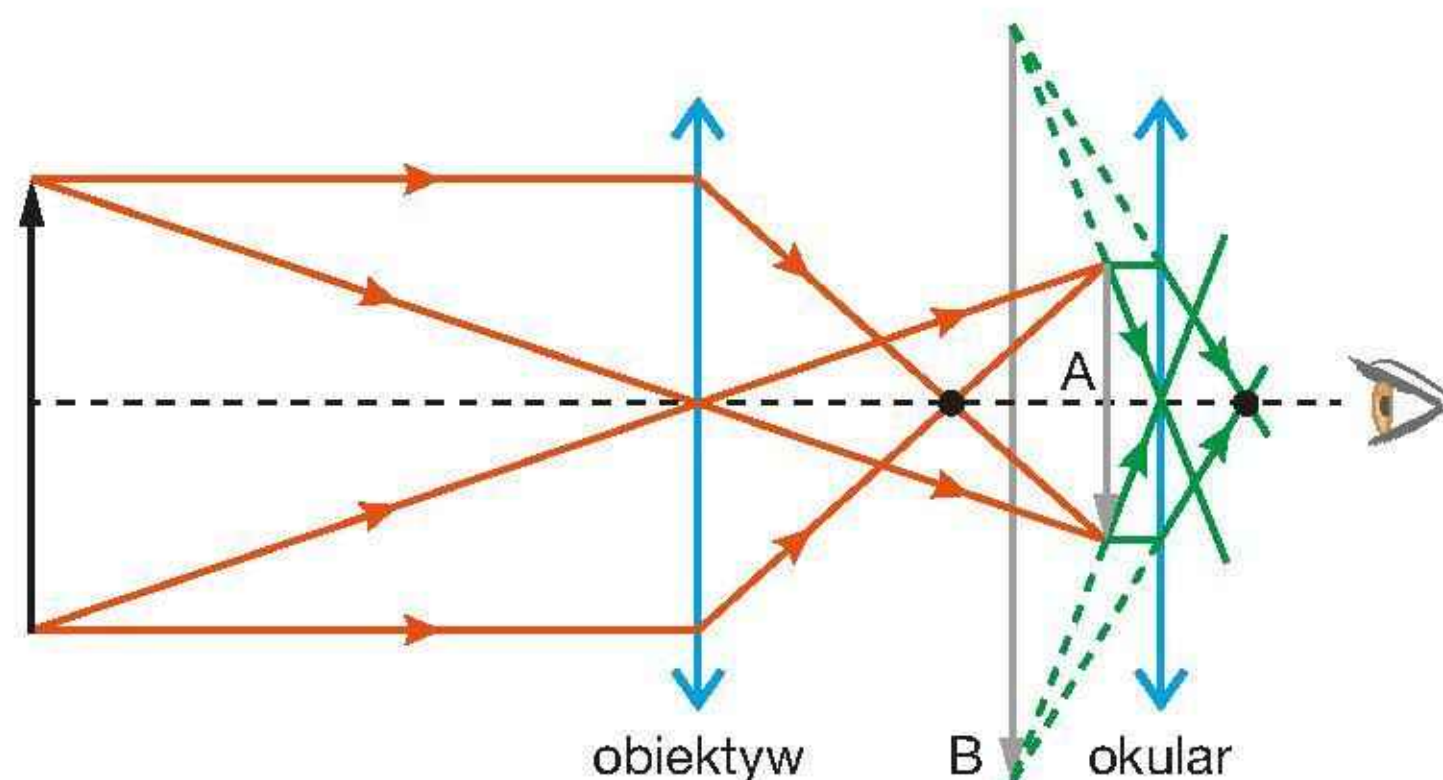
Rys. 16.93. Pierwsza soczewka (obiektyw) tworzy obraz A, który oglądamy przez drugą soczewkę (okular), użytą jako lupa. Widzimy powiększony obraz B małego obrazu A
