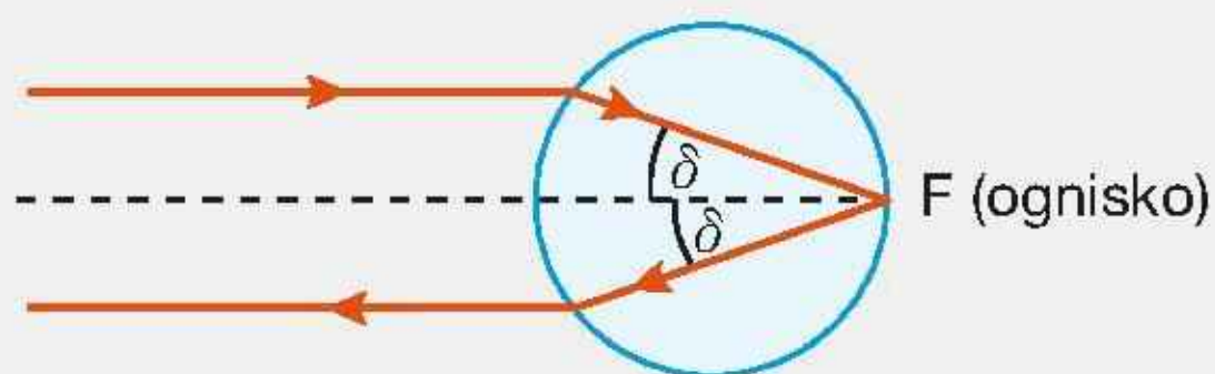
Rys. 2. Odbicie współdrożne w kulce szklanej o współczynniku załamania światła n \approx 2
