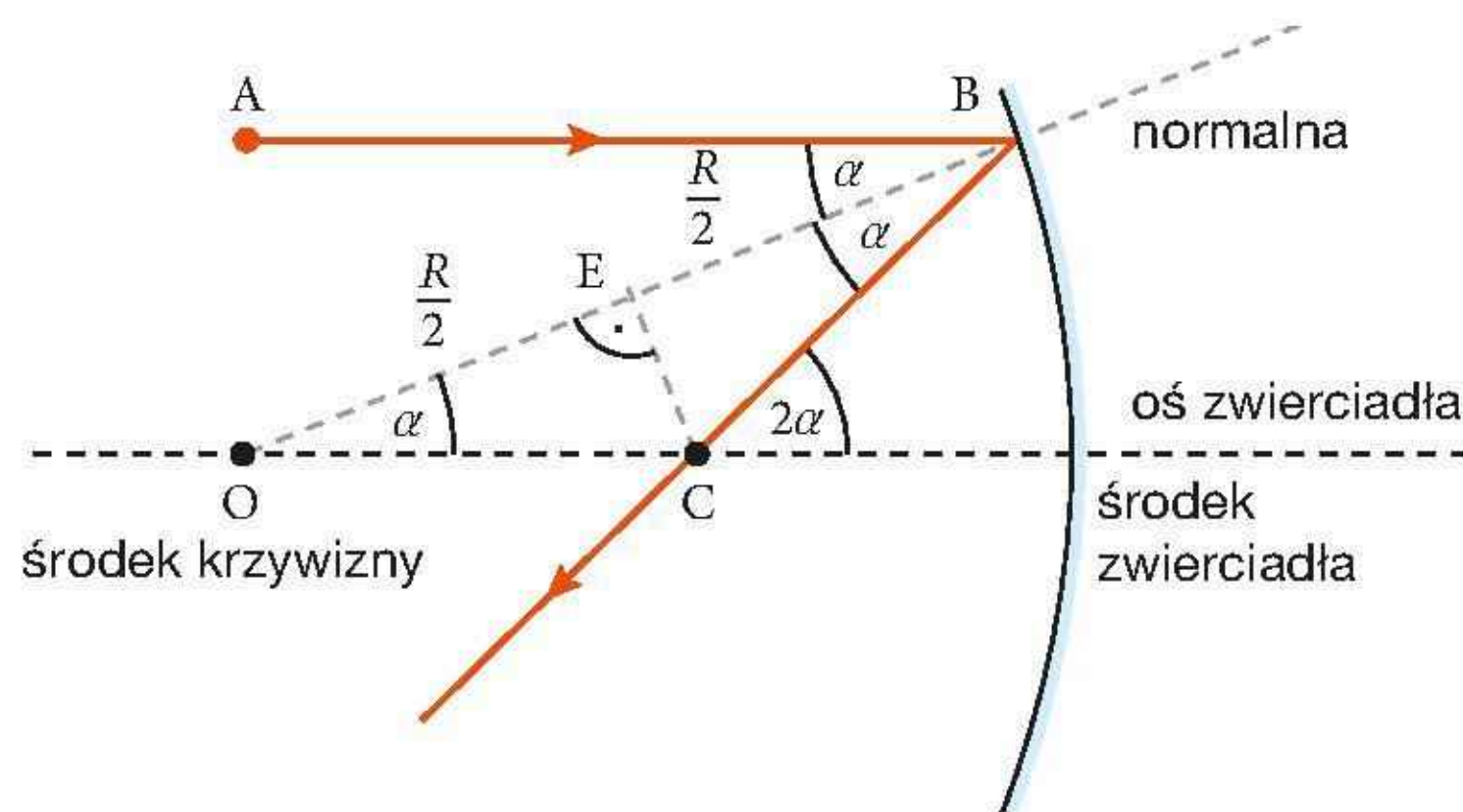
Rys. 16.79. Schemat odbicia promienia równoległego do osi optycznej w zwierciadle wklęsłym
