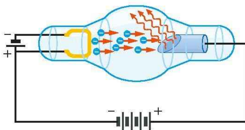
Rys. 17.40. Lampa katodowa wytwarzająca promienie Röntgena
