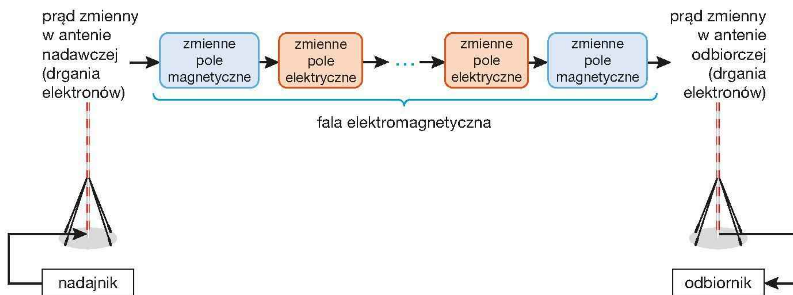
Rys. 16.5. Schemat nadawania i odbierania fal radiowych
