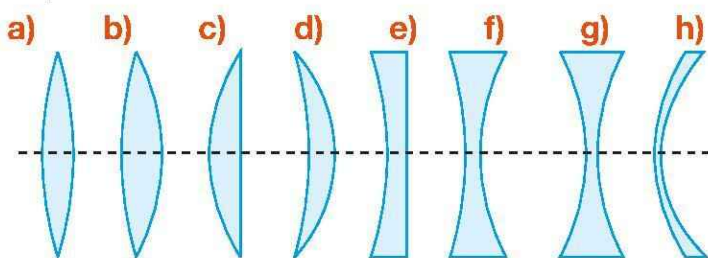
Rys. 16.58. Soczewki o różnych kształtach (widok w przekroju)
