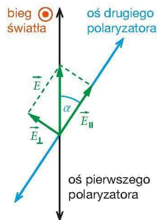
Rys. 16.109. Polaryzacja światła dla polaryzatorów ustawionych pod kątem
