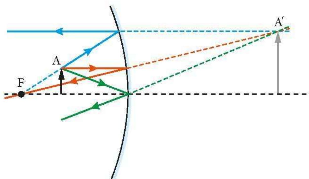
Rys. 16.87. Konstruowanie obrazu tworzonego przez zwierciadło wklęsłe, gdy przedmiot znajduje się bliżej zwierciadła niż ognisko
