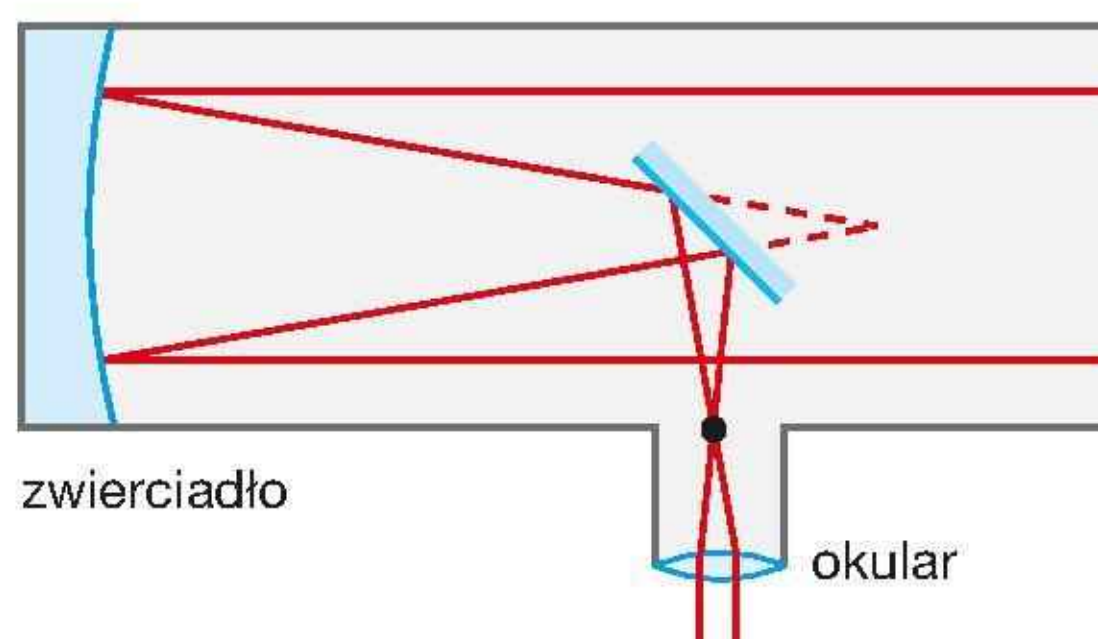
Rys. 16.98. Schemat działania teleskopu zwierciadlanego
