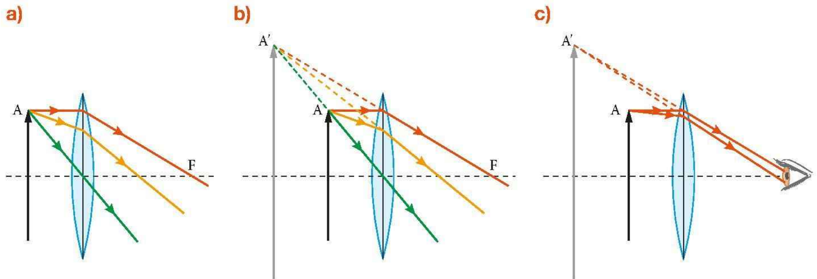
Rys. 16.73. Tworzenie obrazu pozornego przez soczewkę skupiającą, przedmiot znajduje się w odległości mniejszej niż ogniskowa soczewki
