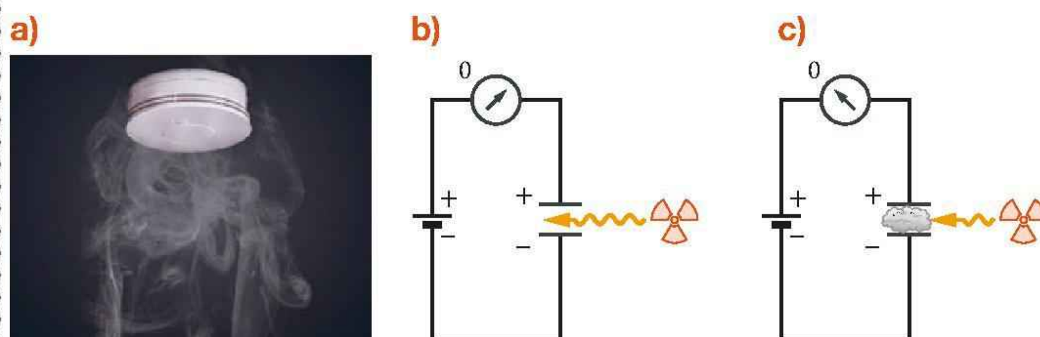
Rys. 18.12. Izotopowy czujnik dymu: a) zdjęcie, b) nie ma dymu – prąd płynie, c) jest dym – natężenie prądu maleje, włącza się alarm
