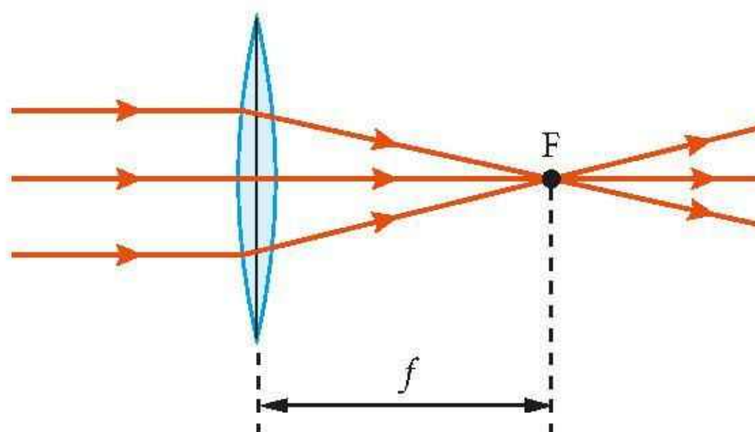
Rys. 16.60. Ognisko i ogniskowa soczewki skupiającej
