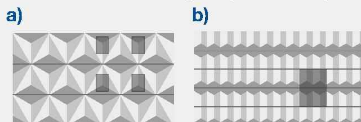
Rys. 4. Schemat budowy pryzmatycznych folii odbłaskowych: (a) standardowa folia mikropryzmatyczna z zaznaczonymi czterema obszarami o maksymalnym odbiciu współdrożnym, (b) 3M Diamond Grade Cubed (DG3)
