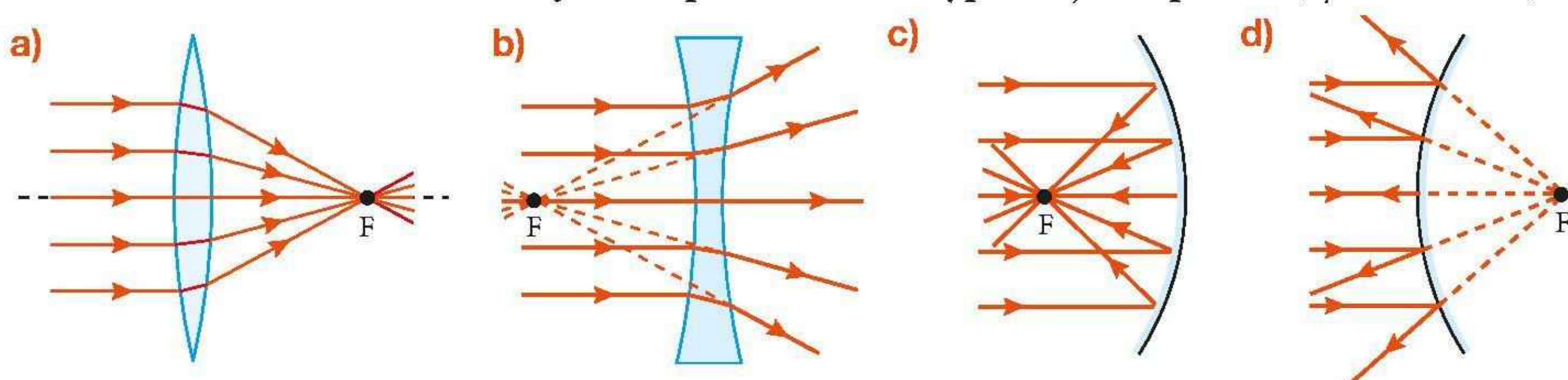
Rys. 16.92. Schematy biegu promieni przechodzących przez różne soczewki i padających na różne zwierciadła
