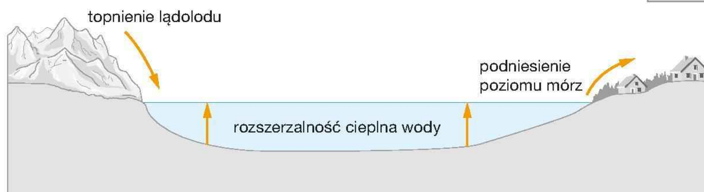
Rys. 17.17. Za wzrost poziomu morza odpowiadają w równym stopniu zwiększająca się ilość wody i jej rozszerzanie się pod wpływem rosnącej temperatury. Słona woda rozszerza się wraz ze wzrostem temperatury zawsze, także poniżej 4°C
