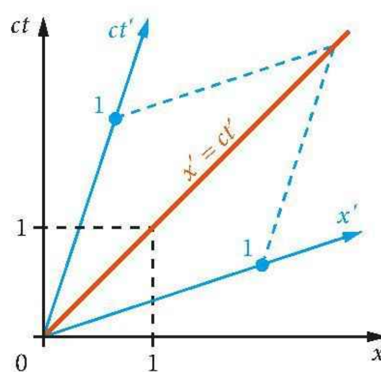
Rys. 19.14. Bieg promienia światła (czerwony): a) transformacja Galileusza, b) transformacja Lorentza
