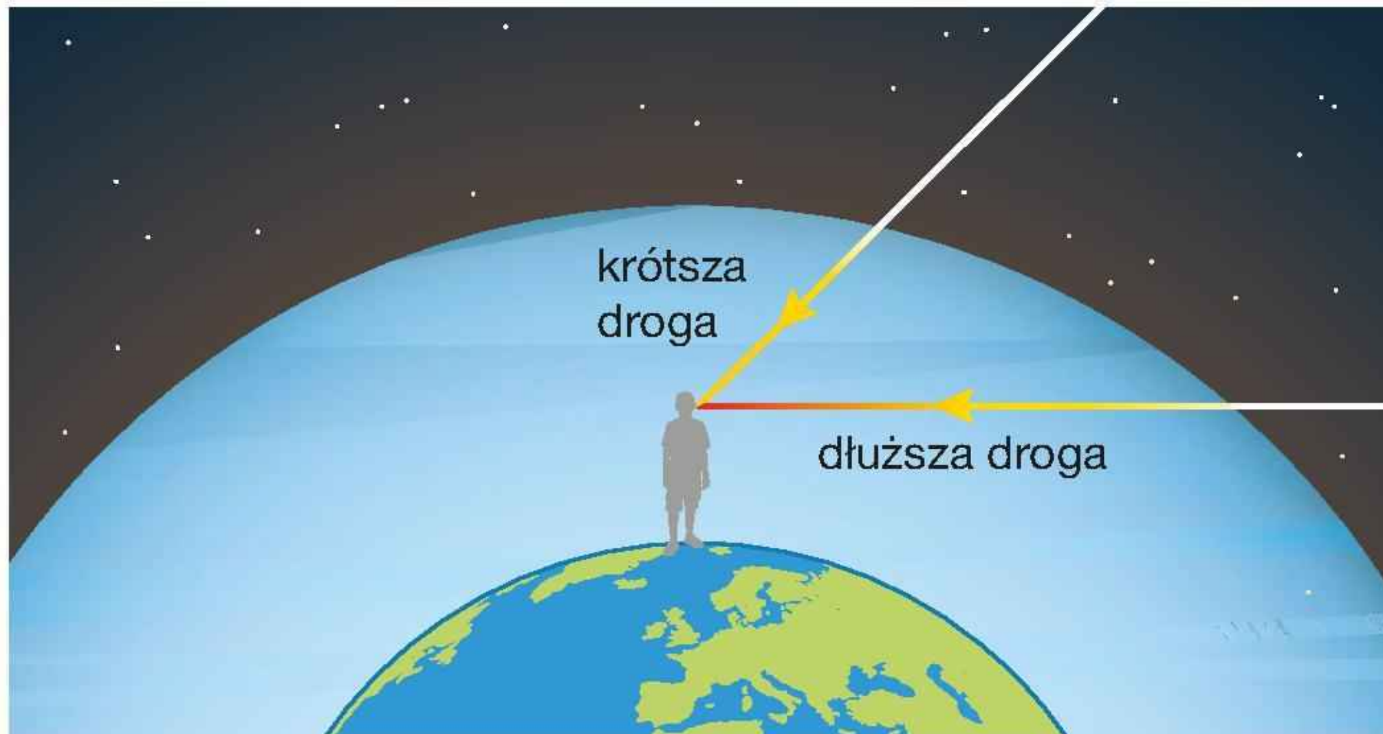
Rys. 16.33. Droga przebyta przez promienie słoneczne w atmosferze zależy od wysokości Słońca nad horyzontem
