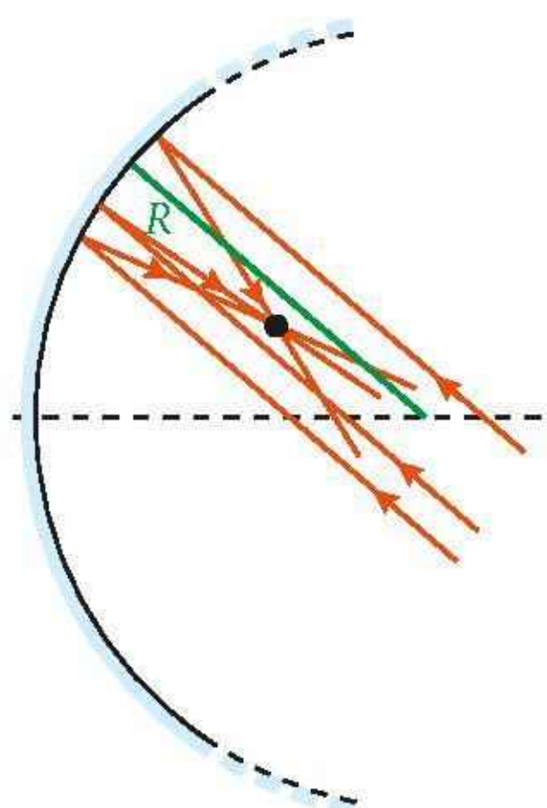
Rys. 16.81. Z zwierciadło sferyczne skupia wąską wiązkę biegnącą wzdłuż promienia niezależnie od kierunku jej padania
