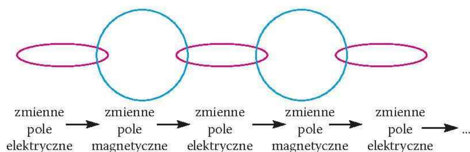
Rys. 16.2. Schemat powstawania fali elektromagnetycznej
