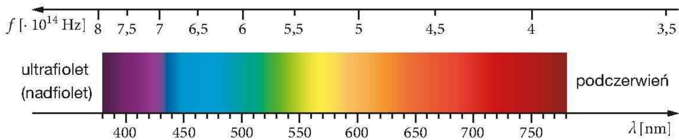
Rys. 16.8. Widmo fal widzialnych ( \lambda – długość fali w próżni)
