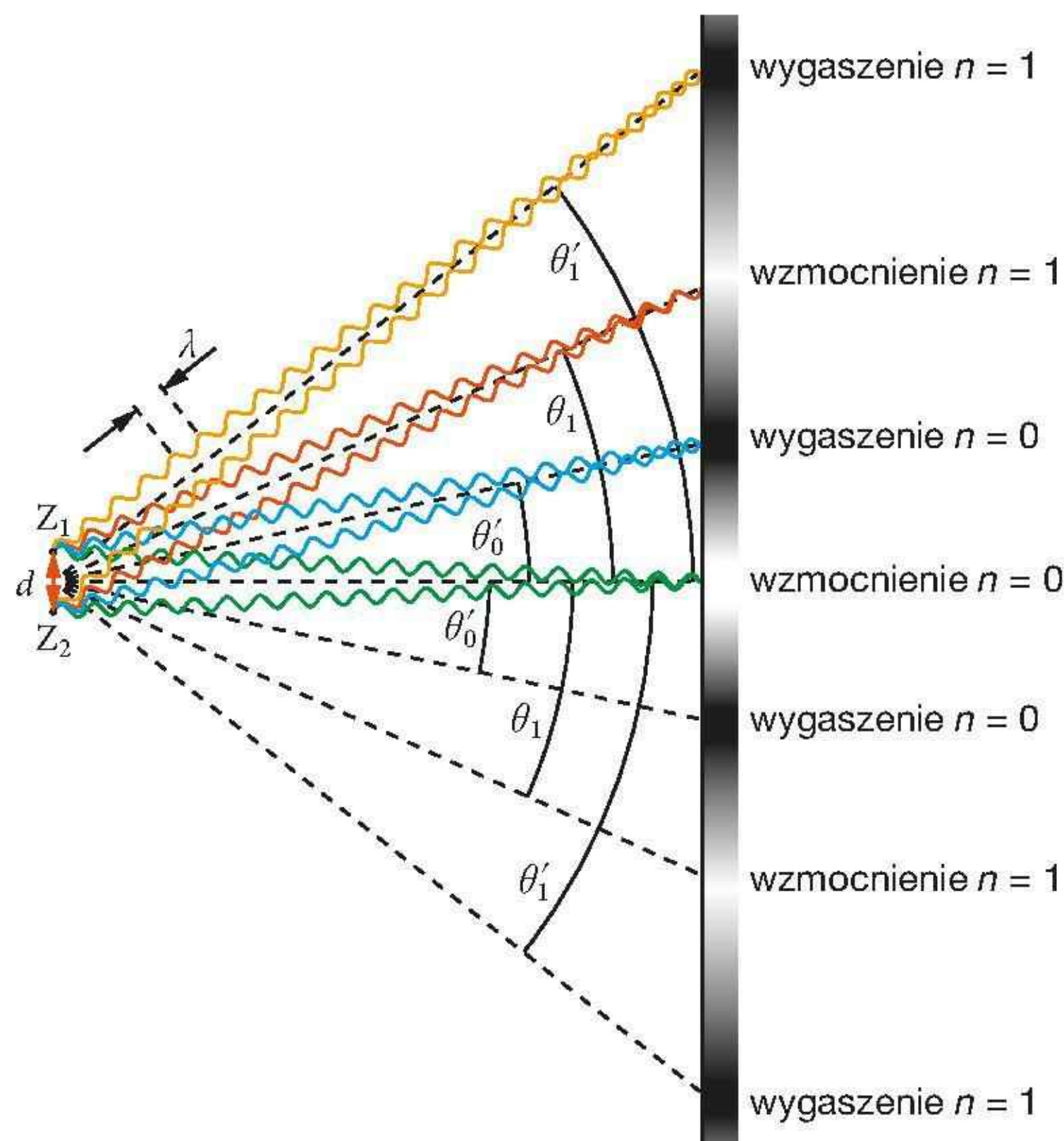
Rys. 16.19. Interferencja fal z dwóch źródeł, widoczne miejsca wzmocnień i wygaszeń fal
