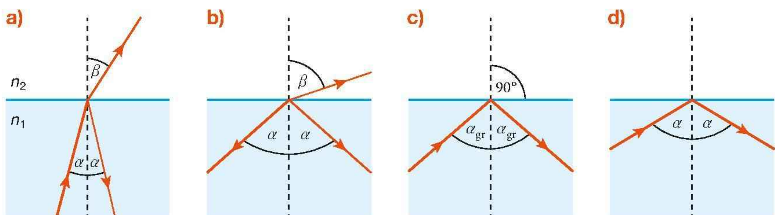
Rys. 16.45. Odbicie wewnętrzne: a) i b) częściowe, c) i d) całkowite
