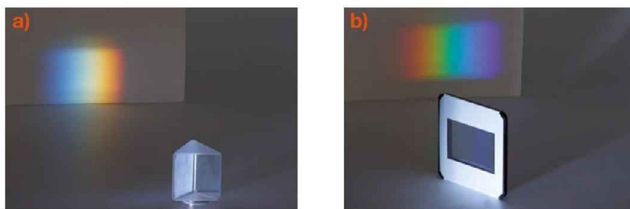
Rys. 16.51. Pryzmat (a) i siatkę dyfrakcyjną (b) oświetlono z tej samej strony. Zwróć uwagę, że mimo to kolory tęczy są w nich ułożone odwrotnie
