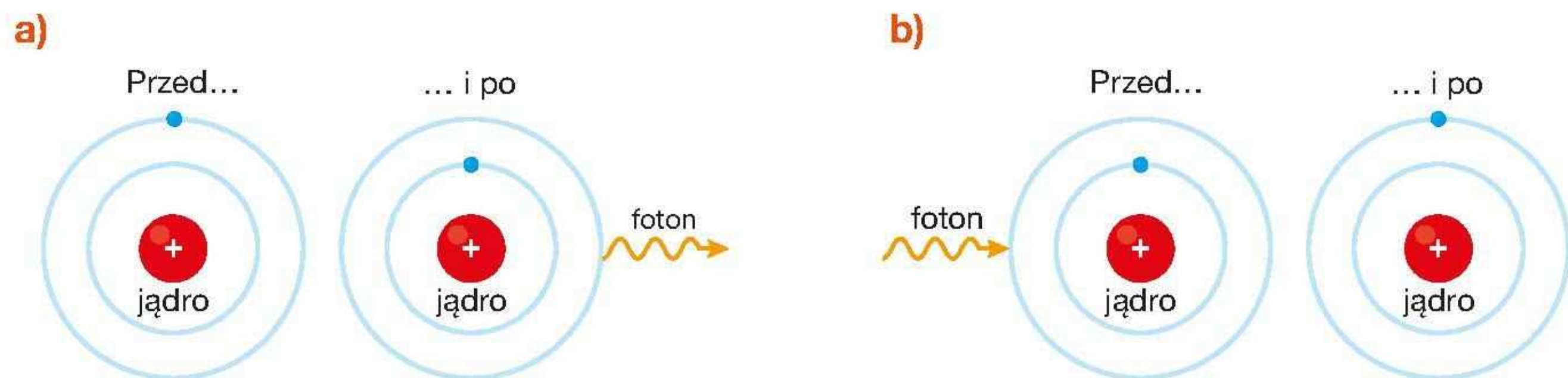
Rys. 17.32. a) wysyłanie (emisja) fotonu, b) pochłanianie (absorpcja) fotonu
