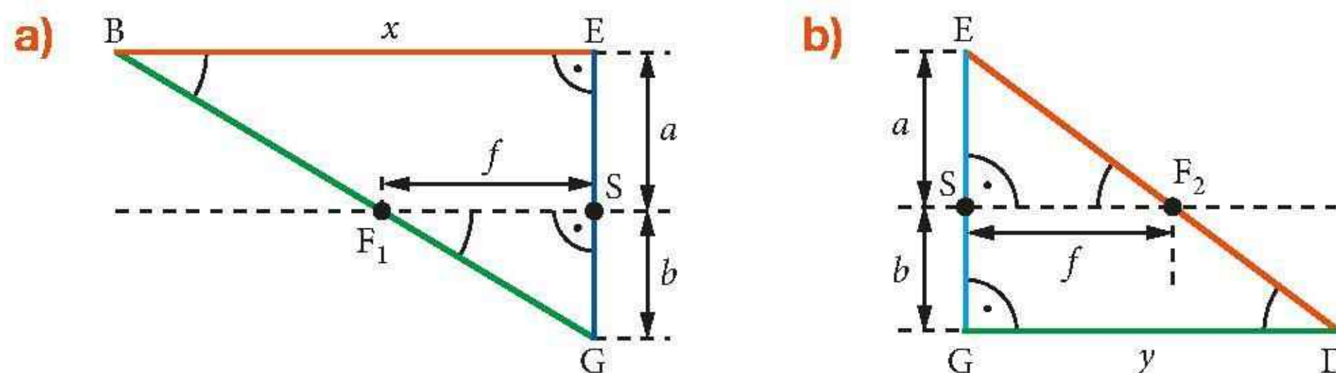
Rys. 16.71. Trójkąty BEG, F_1SG , EGD i ESF_2 z oznaczeniami
