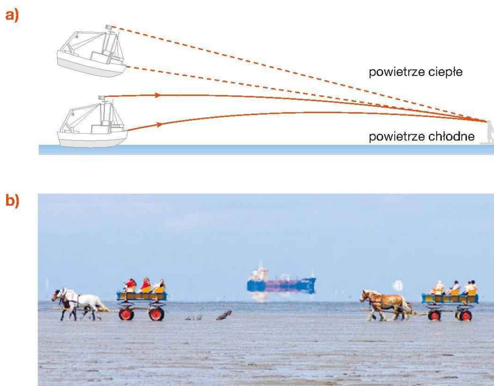
Rys. 16.44. Miraż górny: a) schemat powstawania, b) zjawisko widziane z plaży
