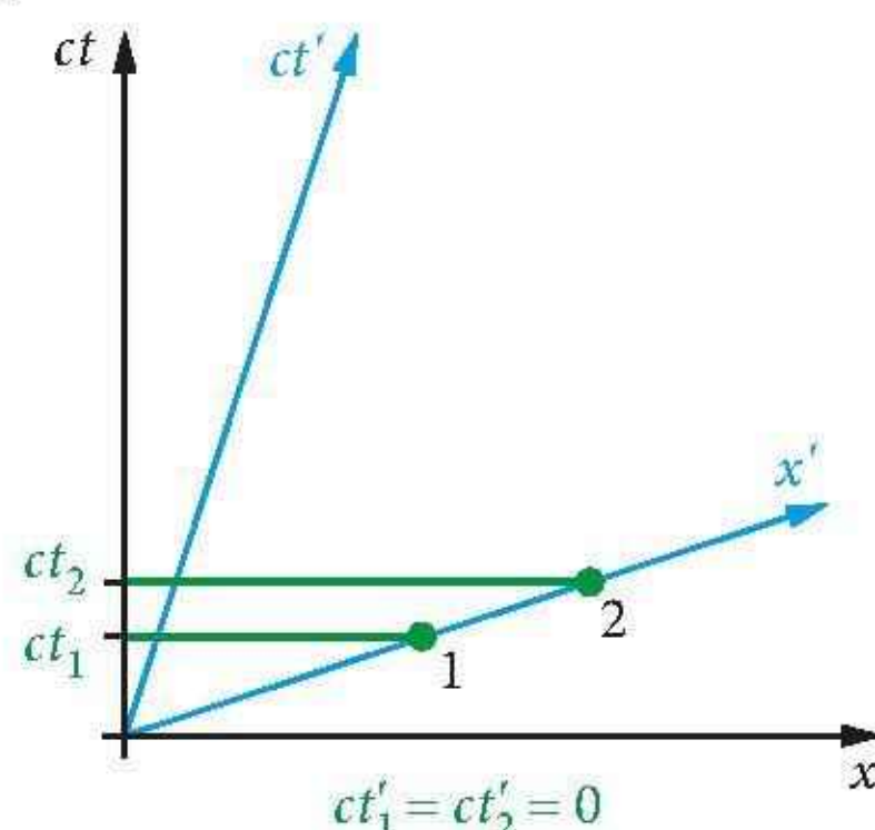
Rys. 19.15. Zdarzenia oznaczone zielonymi kropkami są równoczesne w układzie primowanym, ale nie są równoczesne w układzie nieprimowanym
