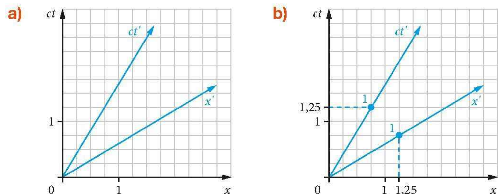
Rys. 19.12. Wyznaczanie układu współrzędnych odpowiadającej transformacji Lorentza dla V = 0,6c : a) kierunek osi, b) jednostka
