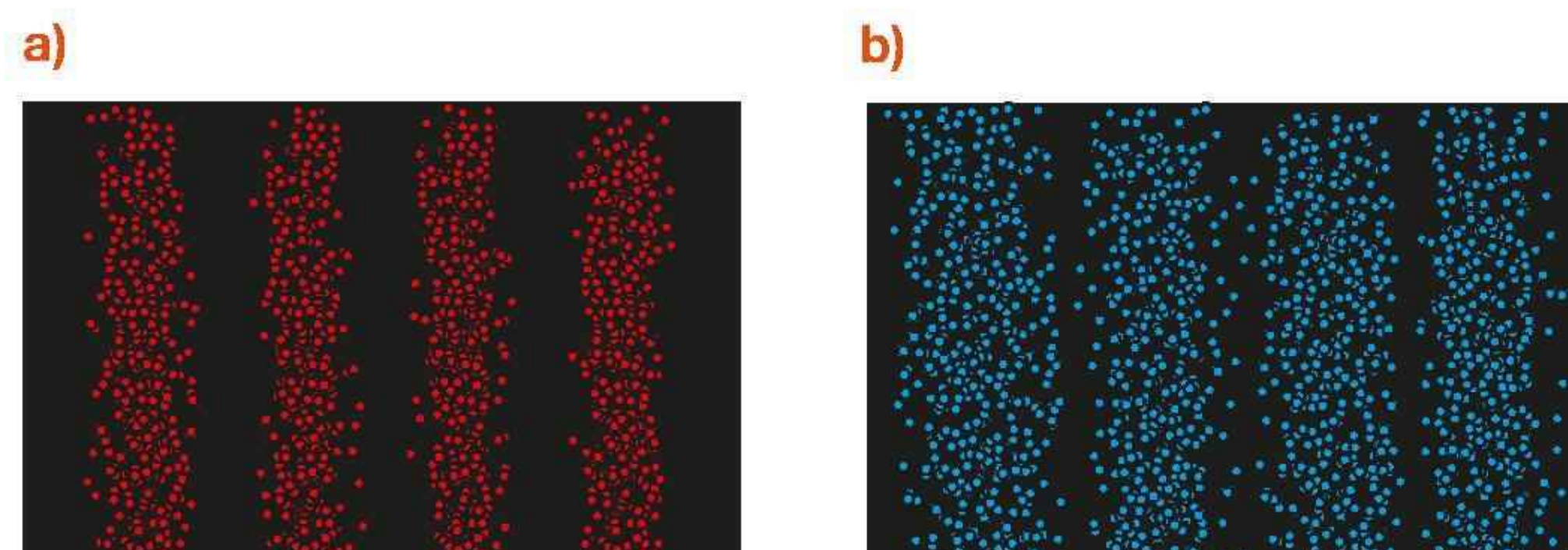
Rys. 17.27. Elektrony (a) i fotony (b) przechodzące przez układ z podwójną szczeliną tworzą bardzo podobne obrazy interferencyjne. Na rysunku przedstawiono wyniki symulacji komputerowej tego zjawiska
