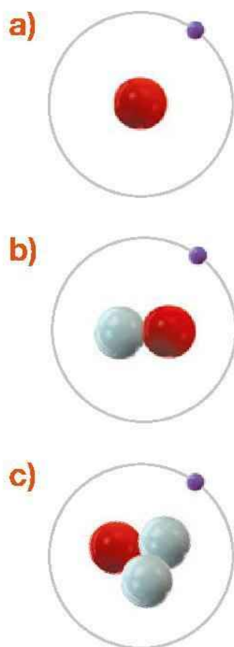
Rys. 18.1. Izotopy wodoru w przyrodzie: a) prot (zwykły wodór) – 99,985%, b) deuter – 0,015%, c) tryt – śladowe ilości
