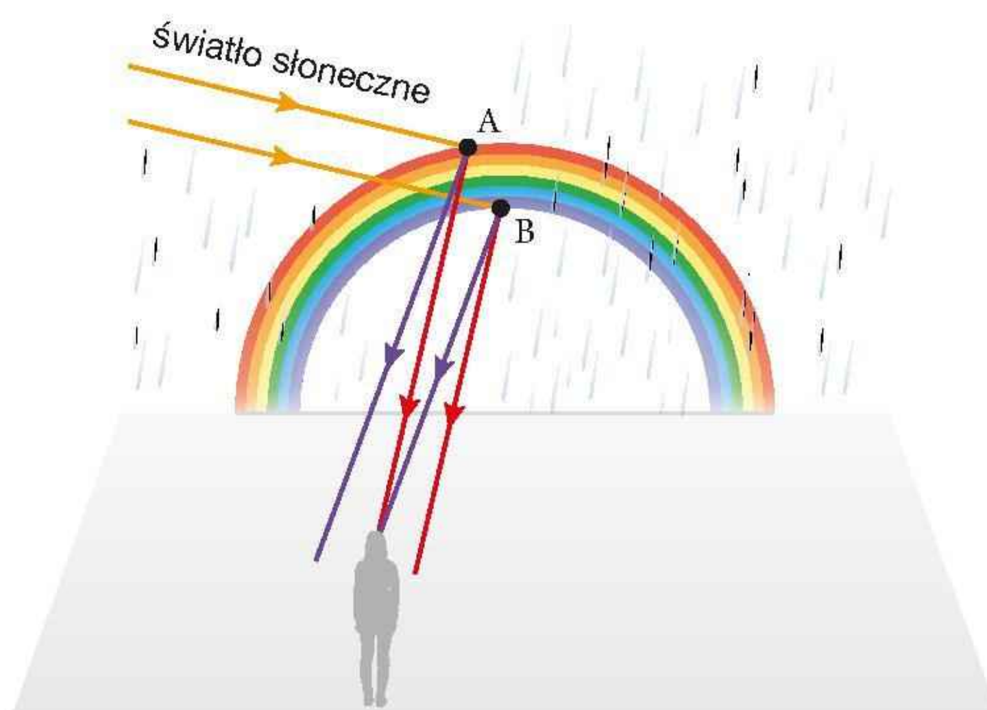
Rys. 16.54. Powstawanie tęczy
