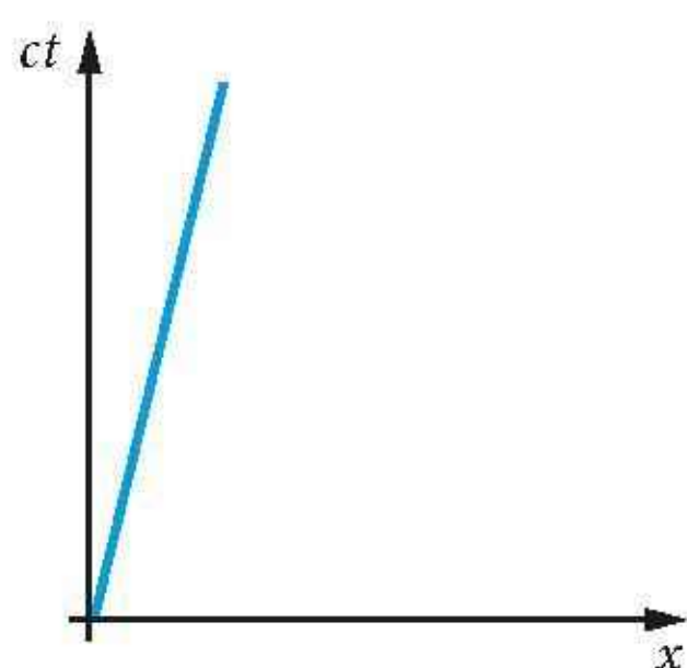
Rys. 19.5. Trajektoria punktu, który w chwili t' = 0 jest w położeniu x' = 0
