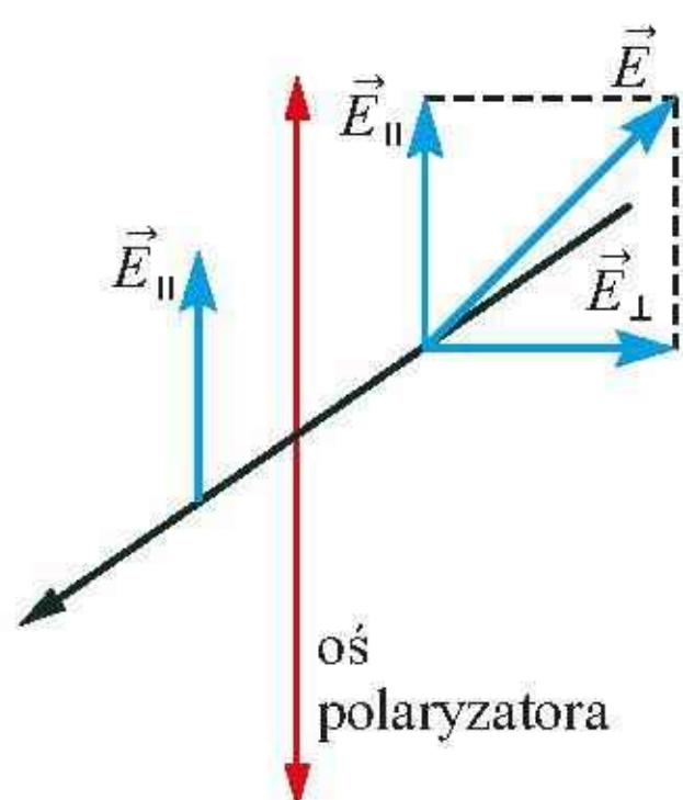
Rys. 16.105. Polaryzator przepuszcza tylko jedną ze składowych wektora natężenia pola elektrycznego \vec{E}
