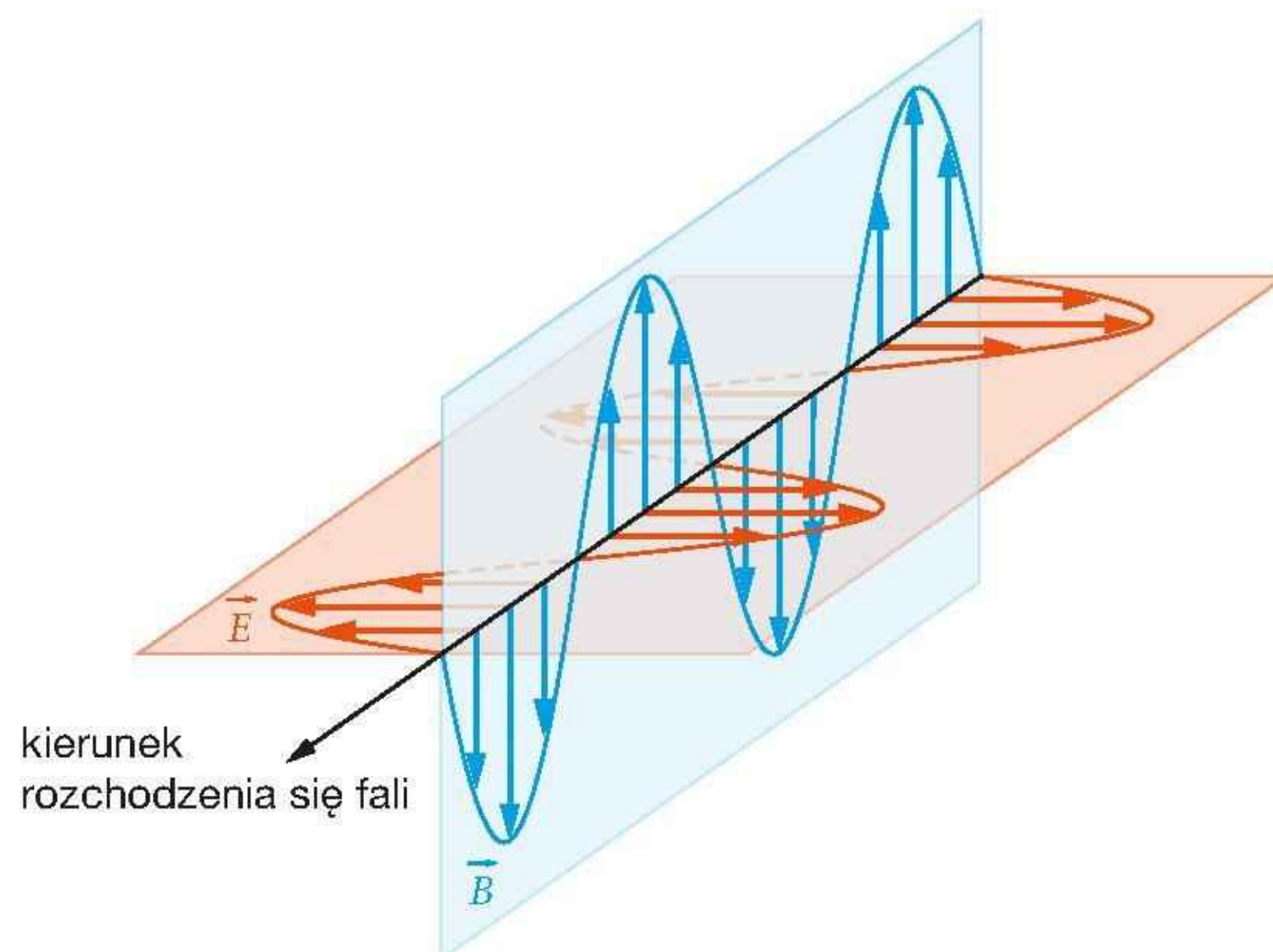
Rys. 16.99. Wektory natężenia pola \vec{E} i indukcji magnetycznej \vec{B} w fali elektromagnetycznej w danej chwili
