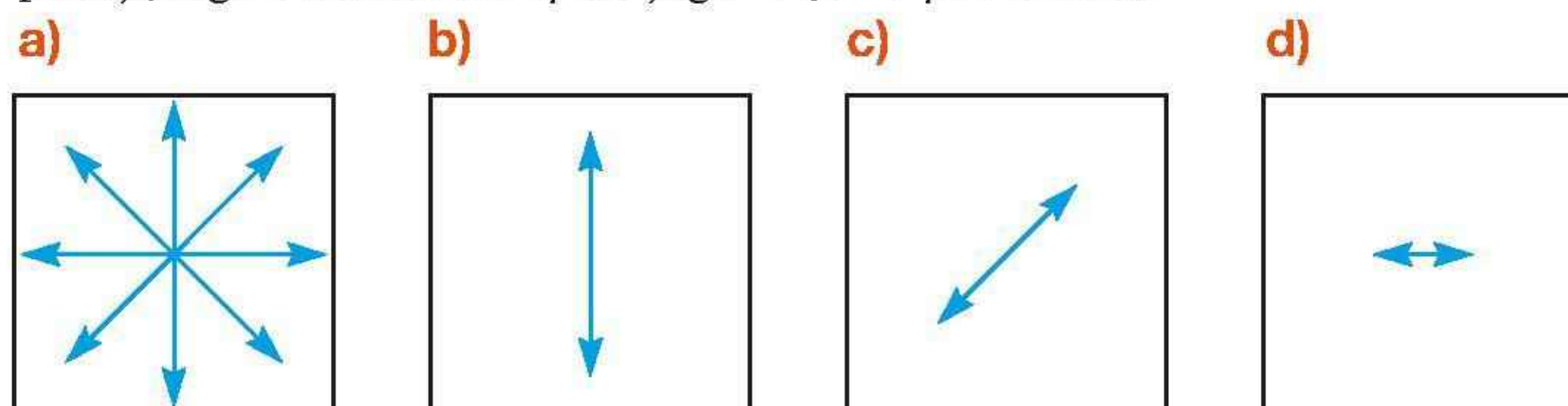
Rys. 16.106. Polaryzacja światła przechodzącego przez trzy polaryzatory (doświadczenie 16. punkt 3): światło niespolaryzowane (a) oraz światło po przejściu przez pierwszy (b), drugi (c) i trzeci (d) polaryzator
