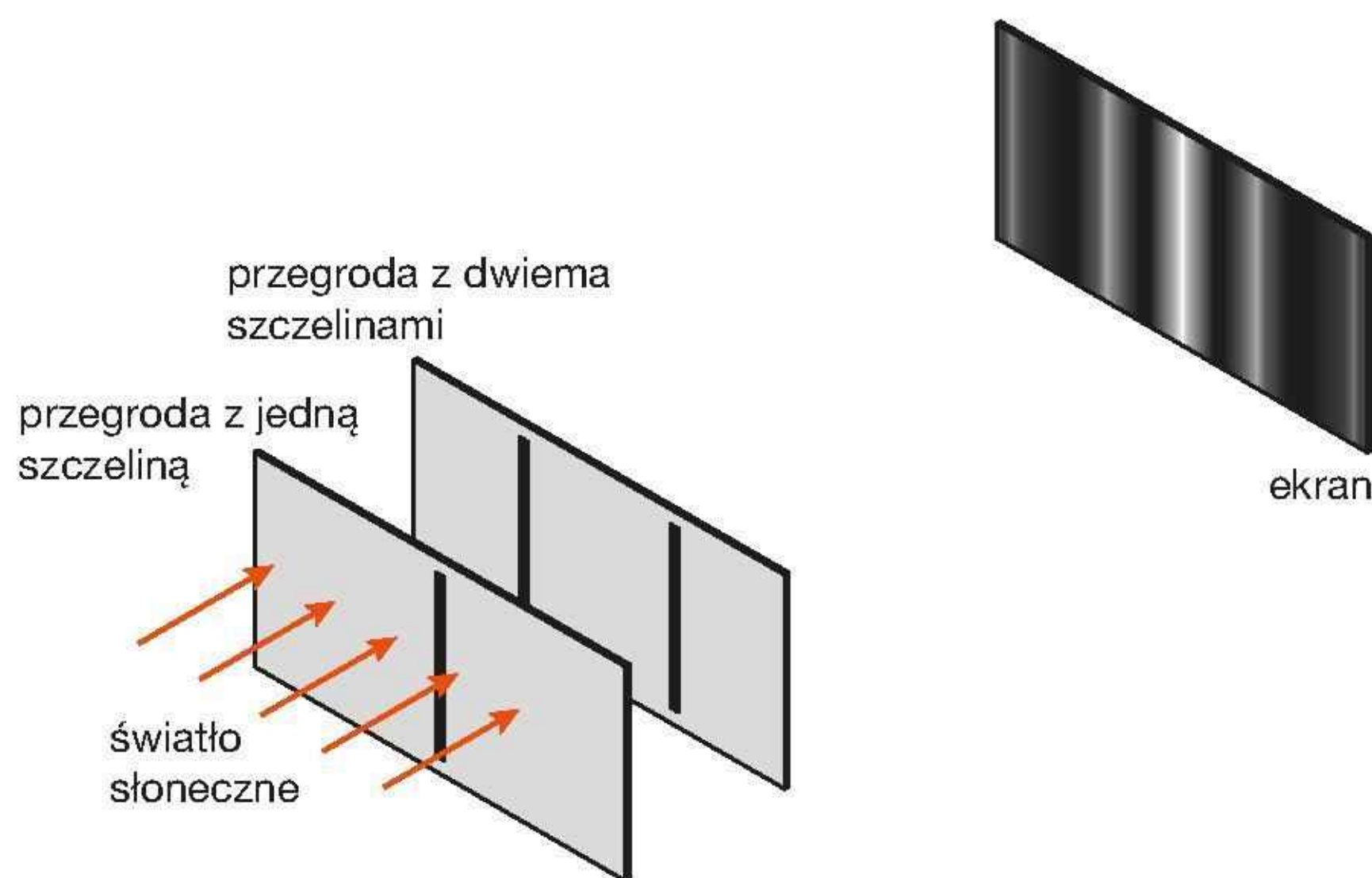
Rys. 16.17. Układ doświadczalny eksperymentu Younga. W rzeczywistości szczeliny w drugiej przegrodzie były bardzo blisko siebie
