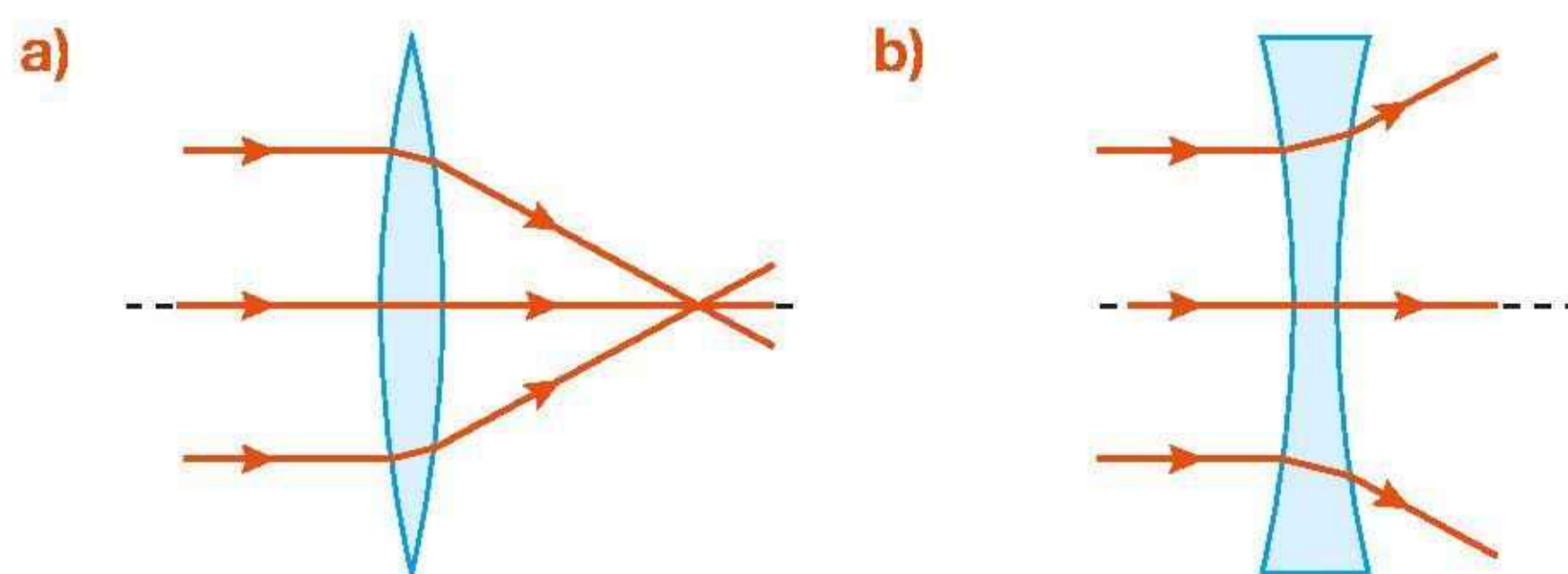
Rys. 16.59. Przejście równoległej wiązki światła przez soczewkę: a) skupiającą, b) rozpraszającą
