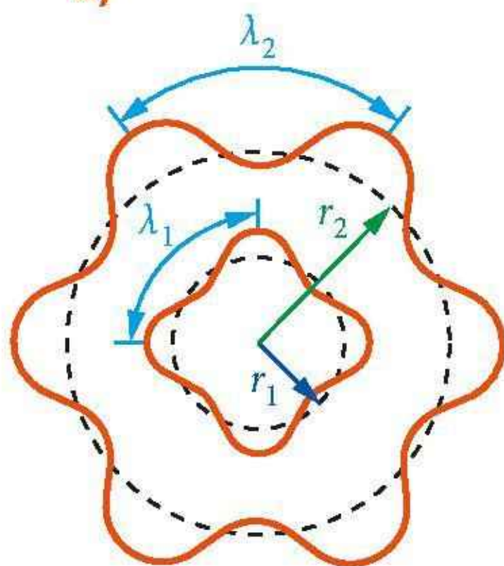
Rys. 17.38. a) przykład fali stojącej na zamkniętej strunie, b) obwód orbity elektronu jest wielokrotnością długości związanej z nim fali materii
