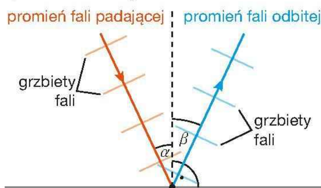
Rys. 16.26. Kąt odbicia \beta jest równy kątowi padania \alpha
