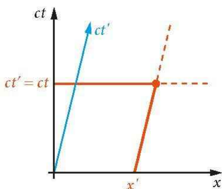
Rys. 19.7. Odczytywanie współrzędnych zdarzenia w układzie wózka (który porusza się z prędkością V )
