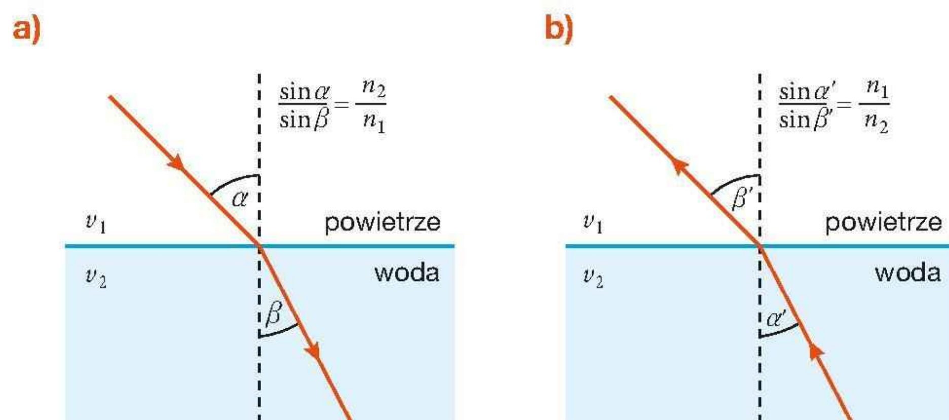
Rys. 16.40. Z powietrza do wody (a) i z wody do powietrza (b) światło może biec po tym samym torze
