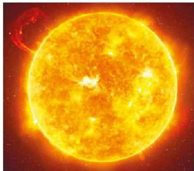
Rys. 18.34. Reakcje termojądrowe w Słońcu zachodzą w jego jądrze
