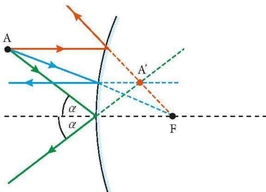
Rys. 16.90. Aby znaleźć obraz punktu w zwierciadle wypukłym, wystarczy prześledzić dwa charakterystyczne promienie
