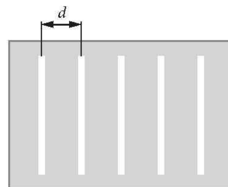
Rys. 16.20. Siatka dyfrakcyjna o pięciu szczelinach
