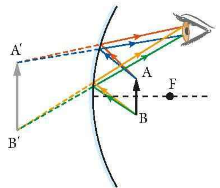
Rys. 16.85. Tworzenie obrazu pozornego przez zwierciadło wklęsłe
