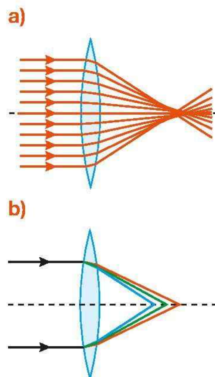
Rys. 16.64. Aberracja a) sferyczna, b) chromatyczna
