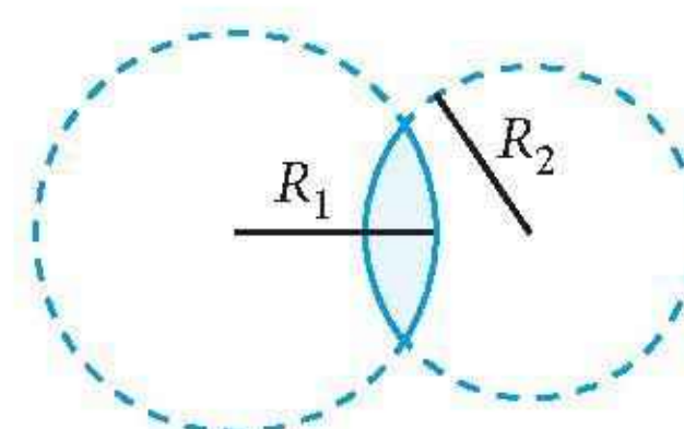
Rys. 16.63. Soczewka sferyczna
