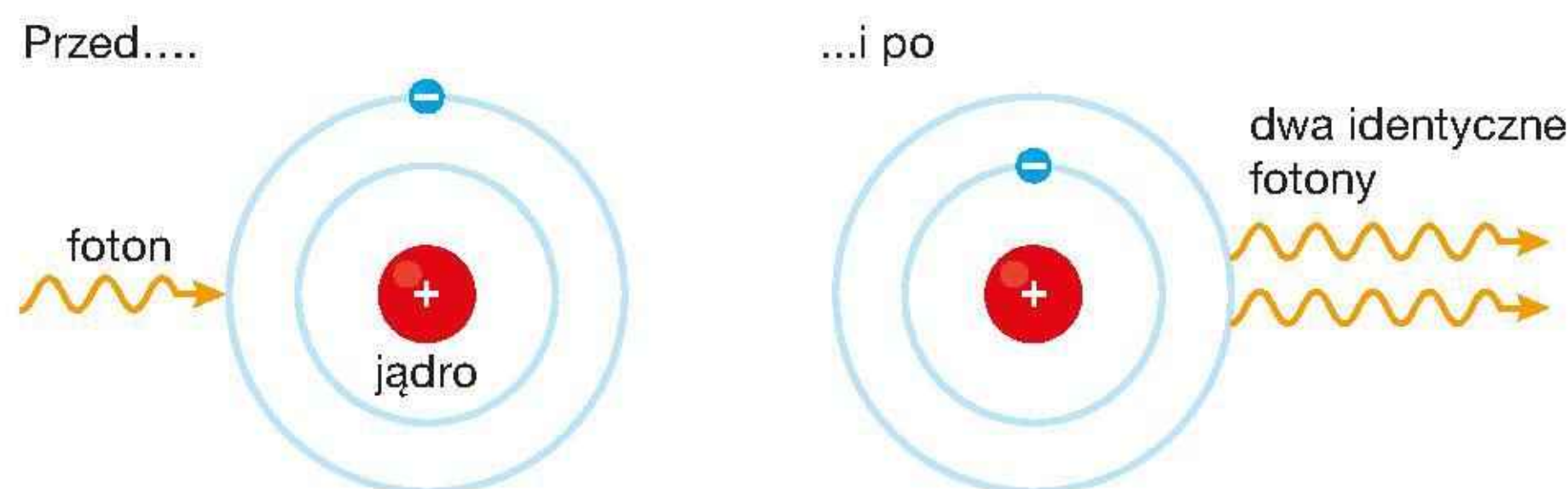
Rys. 17.34. Schemat emisji wymuszonej
