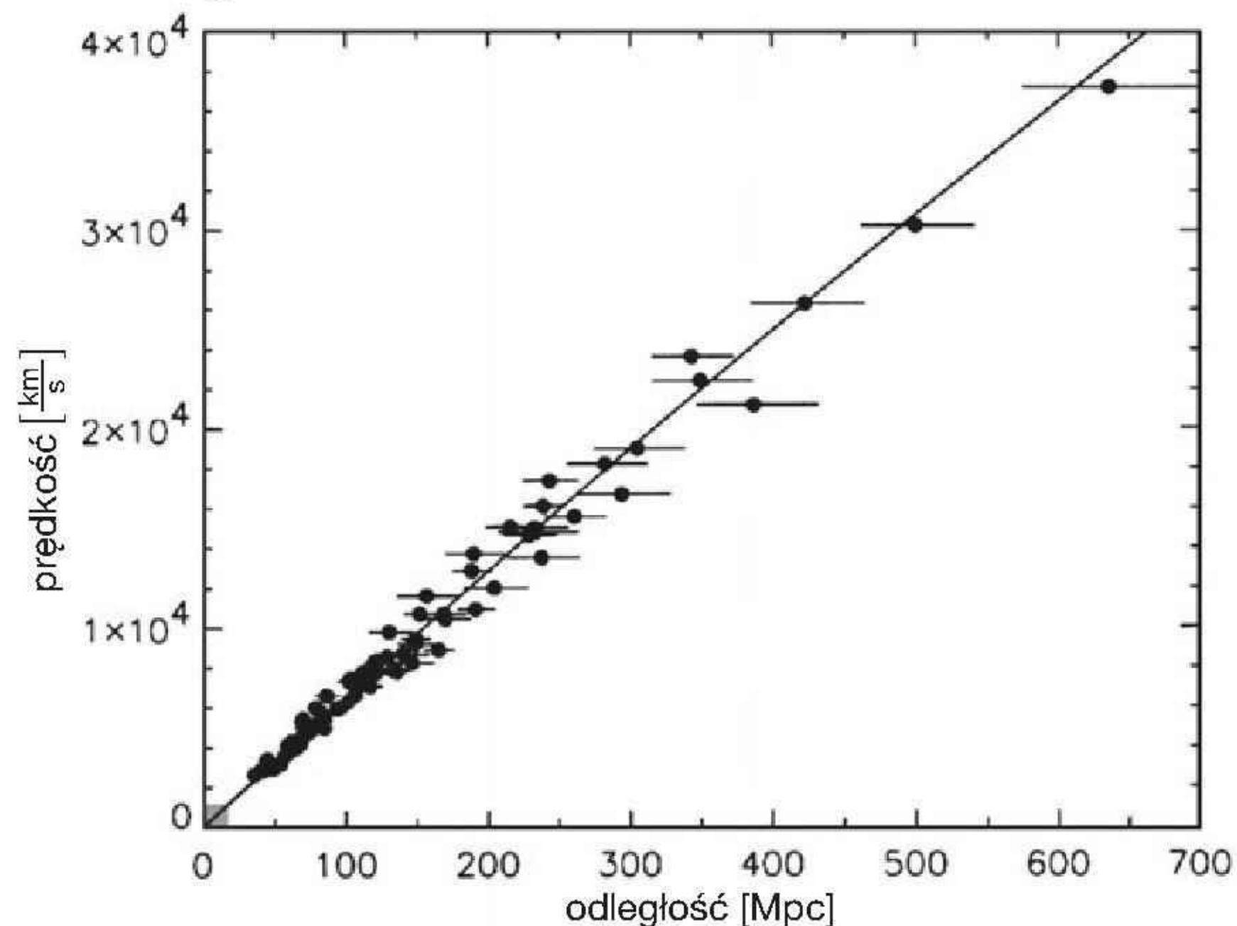
Rys. 18.42. Zależność między odległością do galaktyki a prędkością jej oddalania się od nas
