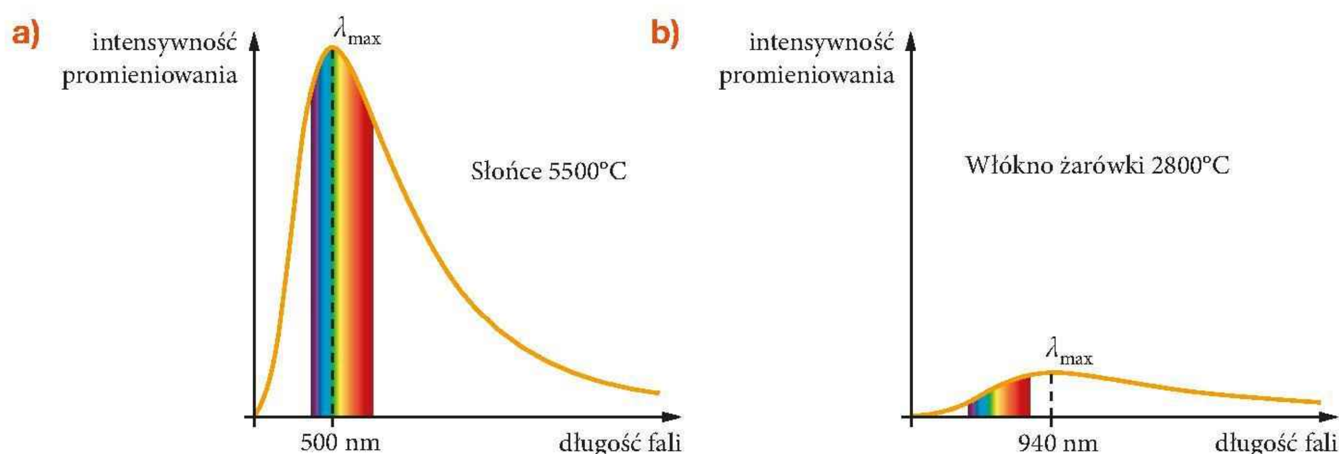
Rys. 17.7. Promieniowanie termiczne Słońca (a) i tradycyjnej żarówki (b)
