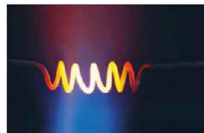
Rys. 17.10. Gołym okiem widzimy, że metalowa spirala jest najbardziej rozgrzana pośrodku
