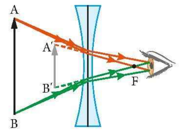
Rys. 16.75. Schemat ilustrujący, w jaki sposób widzimy obraz tworzony przez soczewkę rozpraszającą
