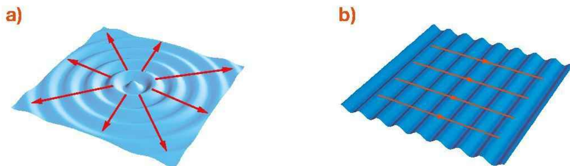
Rys. 16.35. Grzbiety i promienie fal na wodzie (promienie oznaczono czerwonymi strzałkami): a) fala kolista, b) fala płaska
