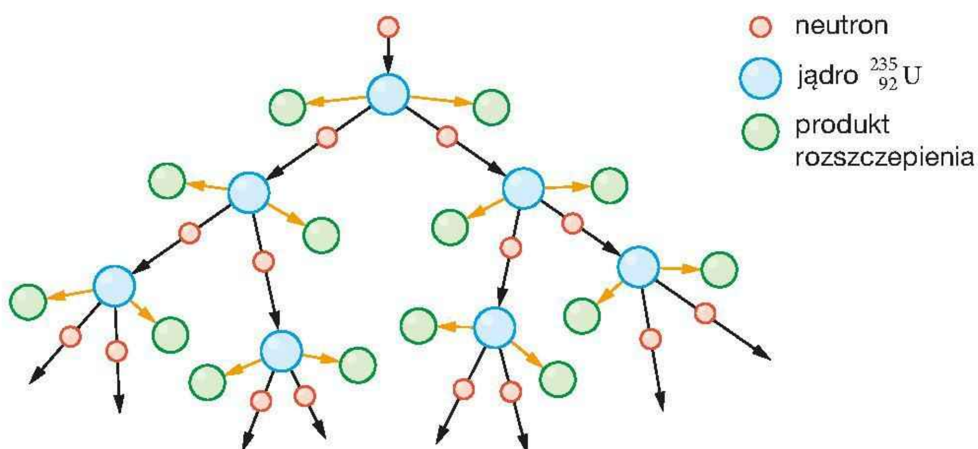
Rys. 18.24. Schemat reakcji łańcuchowej zachodzącej w bryle uranu ^{235}\text{U} (bez zachowania skali). Czarne strzałki przedstawiają tory ruchu neutronów, powodujących rozszczepienie kolejnych jąder uranu
