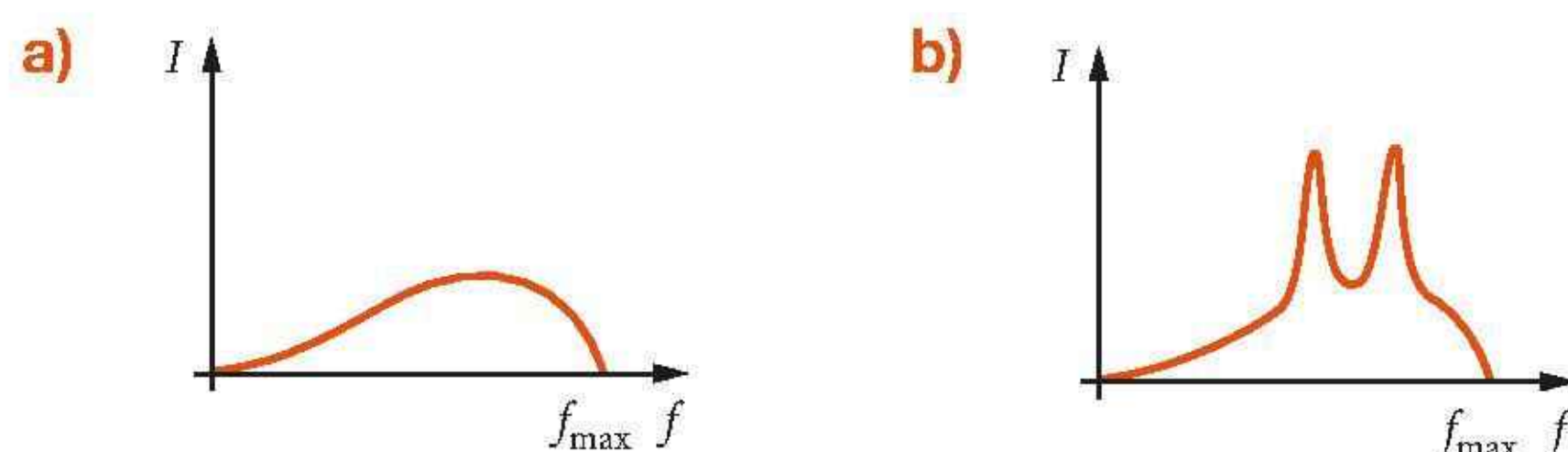
Rys. 17.41. Widmo promieniowania rentgenowskiego: a) promieniowanie hamowania, b) pełny wykres
