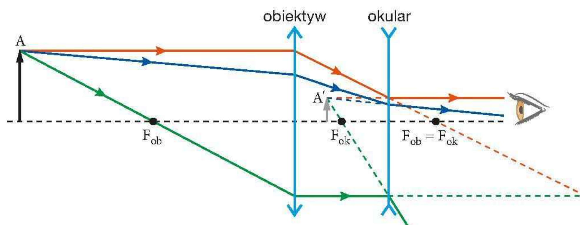
Rys. 16.96. Schemat zasady działania lunety Galileusza
