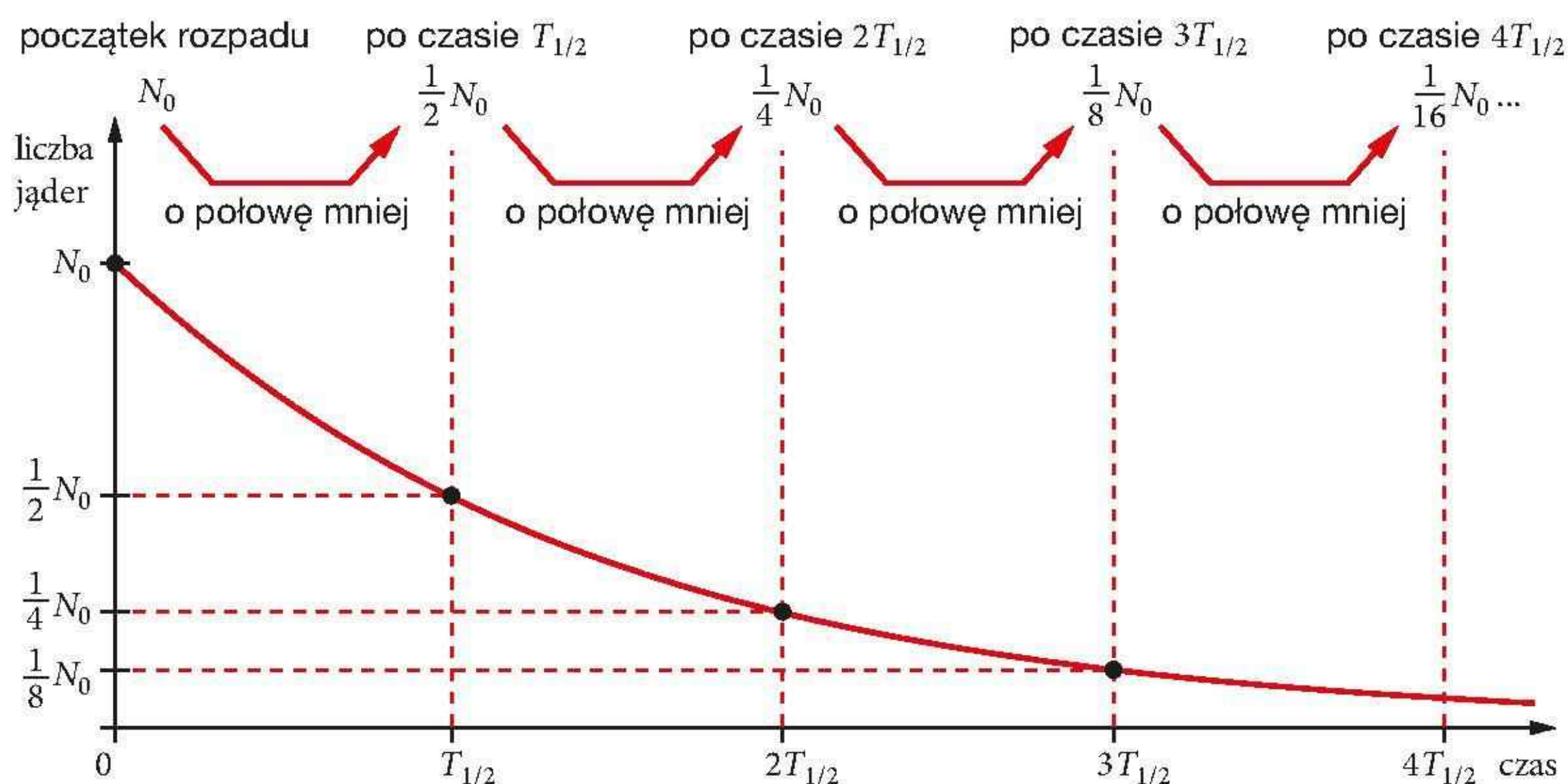
Rys. 18.15. Wykres zależności liczby jąder materialu promieniotwórczego od czasu
