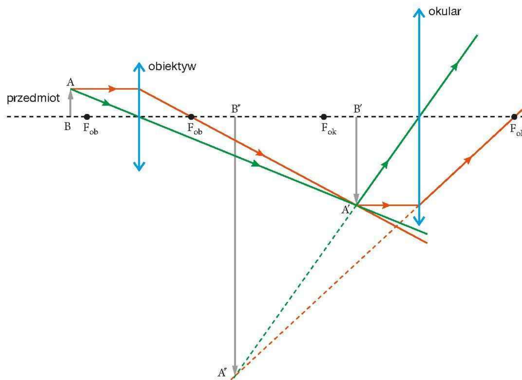
Rys. 16.97. Schemat powstawania obrazu w mikroskopie optycznym
