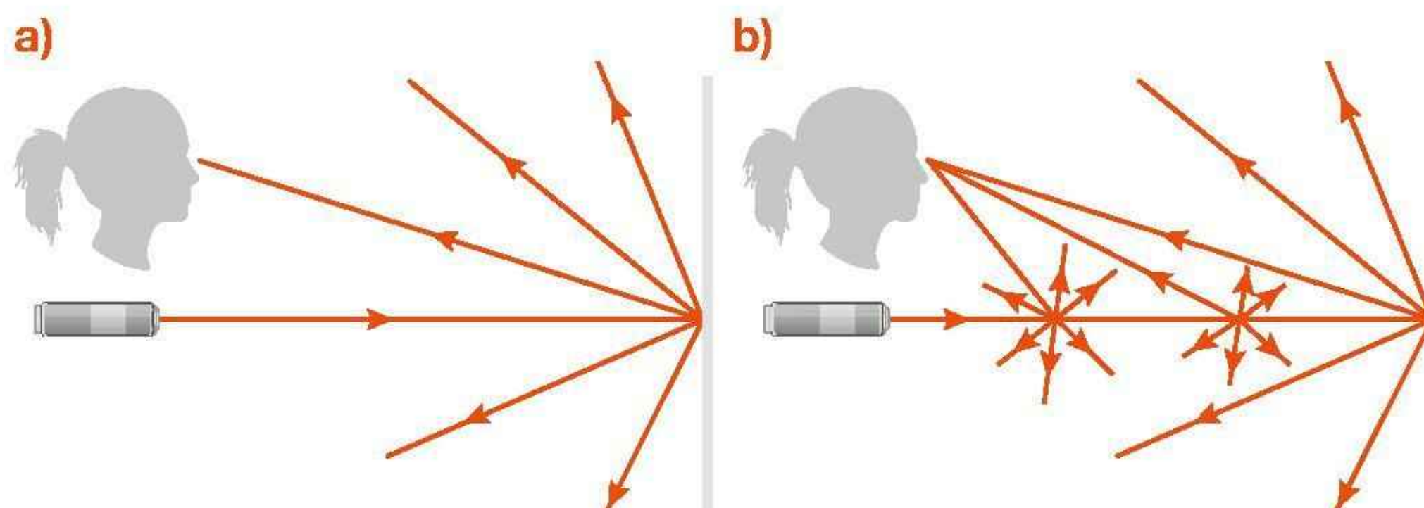
Rys. 16.29. Widoczność wiązki lasera w powietrzu: a) czystym, b) zanieczyszczonym
