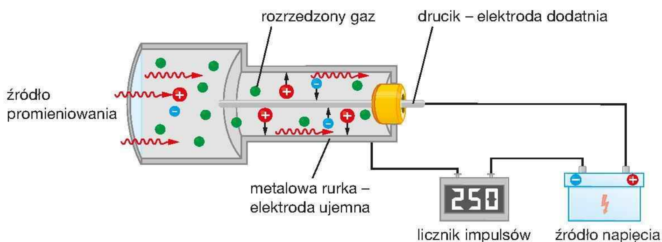
Rys. 18.5. Licznik Geigera–Müllera
