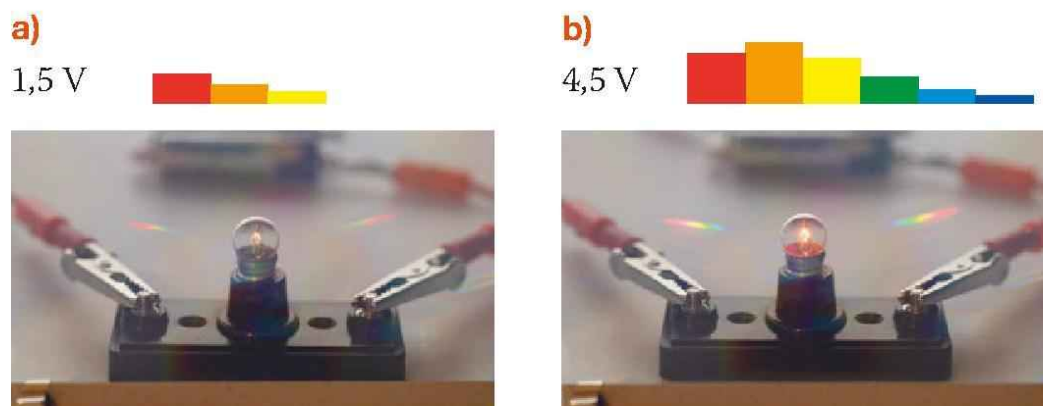
Rys. 17.6. Prawa żarówka emituje więcej światła pomarańczowego niż czerwonego, ale i tak światła czerwonego emituje więcej niż żarówka lewa
