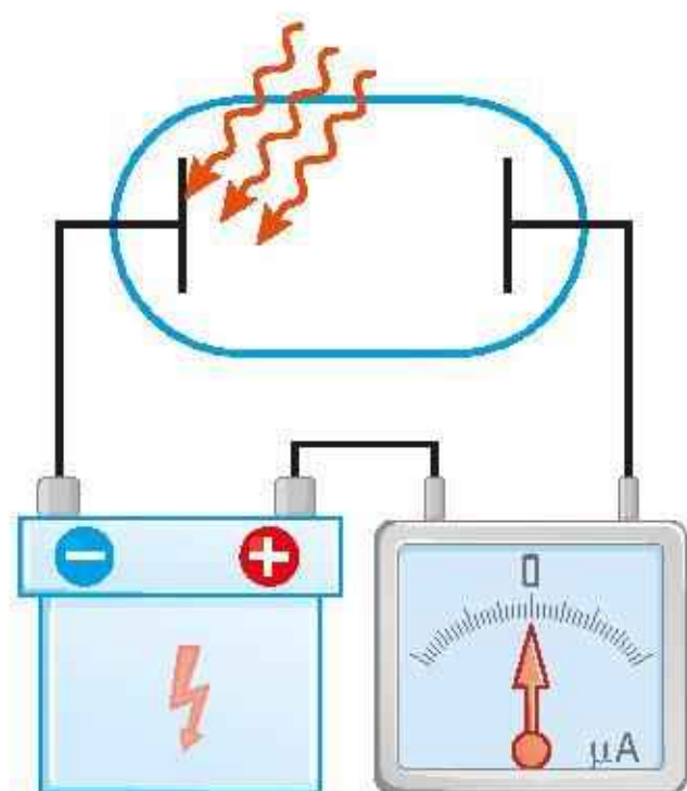
Rys. 17.19. Jeżeli elektrody fotokomórki są zbudowane z cezu, to oświetlenie światłem czerwonym nie powoduje przepływu prądu
