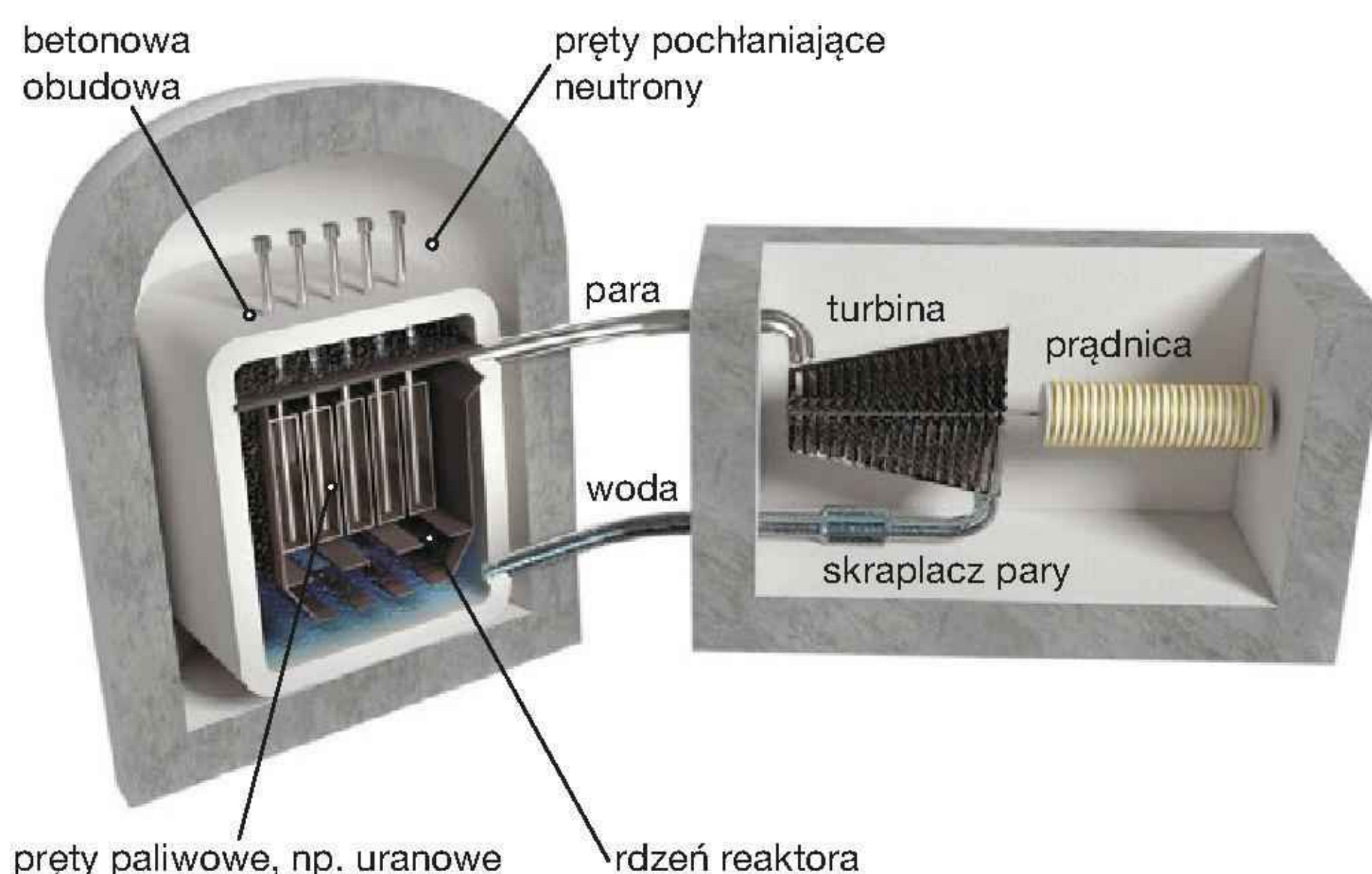
Rys. 18.27. Uproszczony schemat elektrowni jądrowej. Dziś stosuje się konstrukcje bardziej skomplikowane, ale dzięki temu bezpieczniejsze
