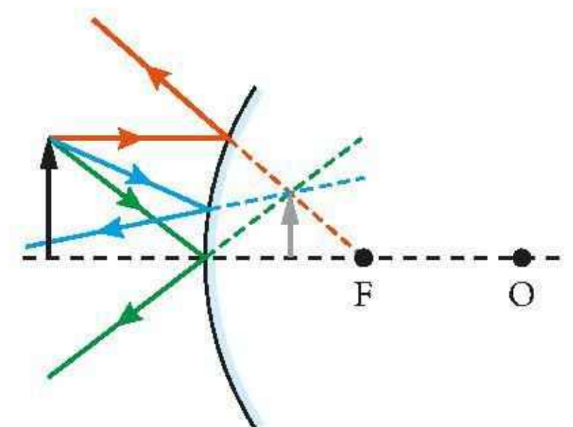
Rys. 16.89. Powstawanie obrazu w zwierciadle wypukłym
