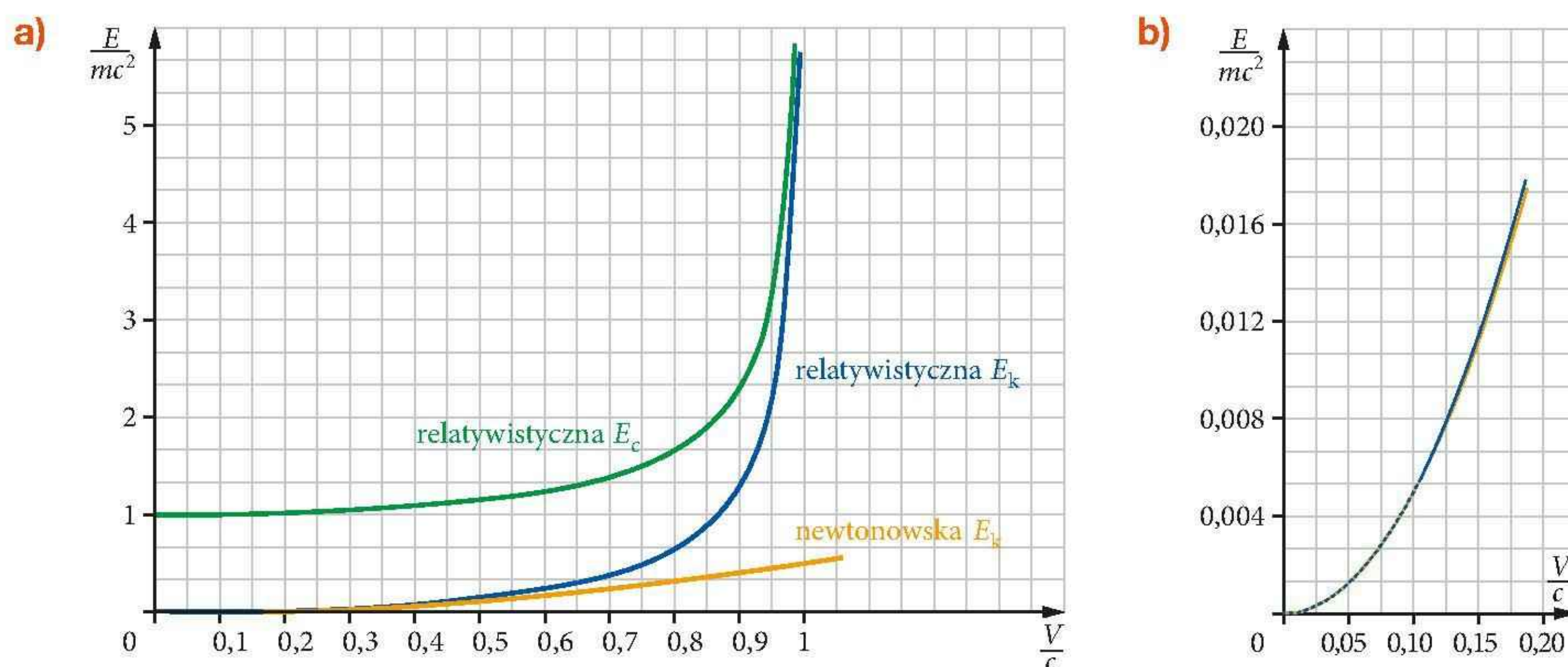
Rys. 19.27. Porównanie zależności energii od prędkości. Na rysunku b) powiększony początkowy obszar wykresu
