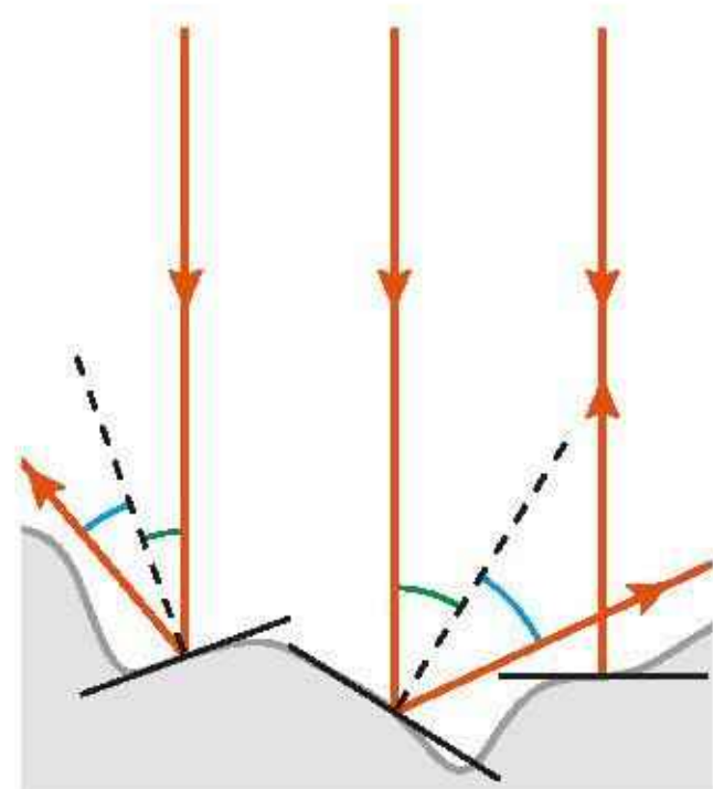
Rys. 16.27. Rozproszenie przy odbiciu od nieregularnej powierzchni
