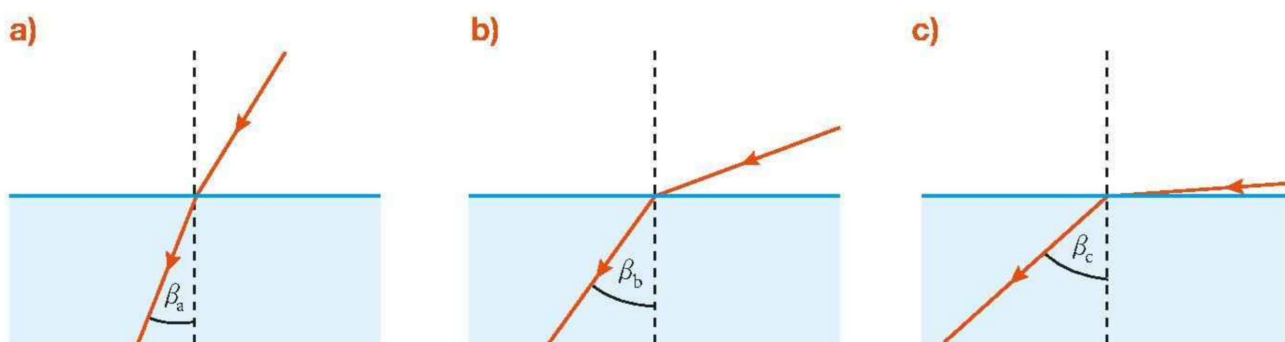
Rys. 16.48. Załamanie promieni światła padających z powietrza do wody pod różnymi kątami
