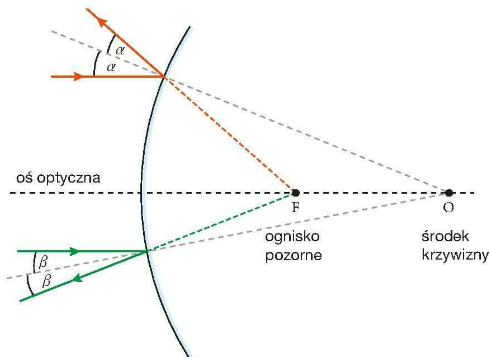
Rys. 16.88. Zwierciadło wypukłe rozprasza wiązkę światła (zaznaczono dwa skrajne promienie)
