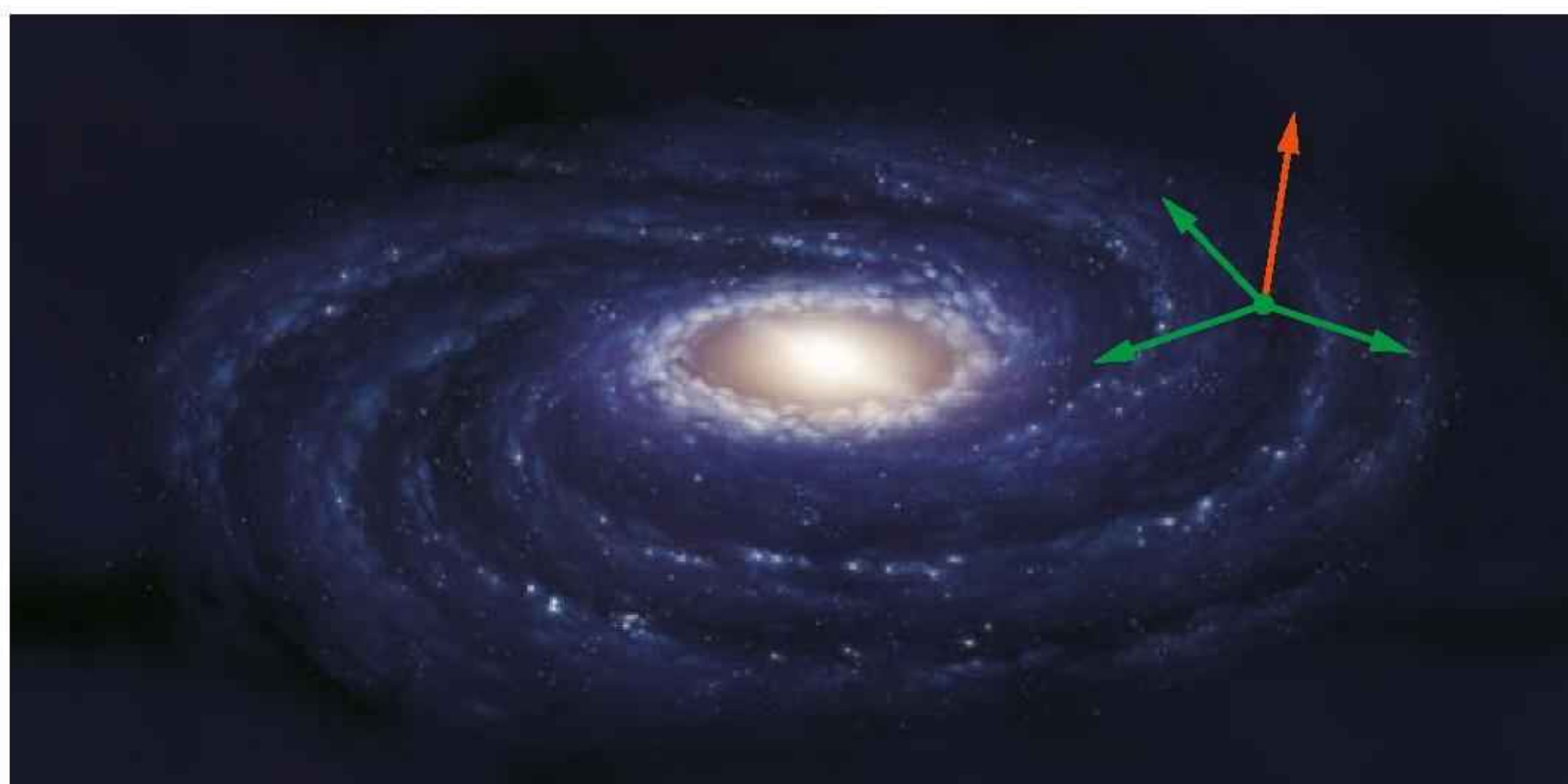
Rys. 18.40. Jak powstaje obraz Galaktyki z jej wnętrza
