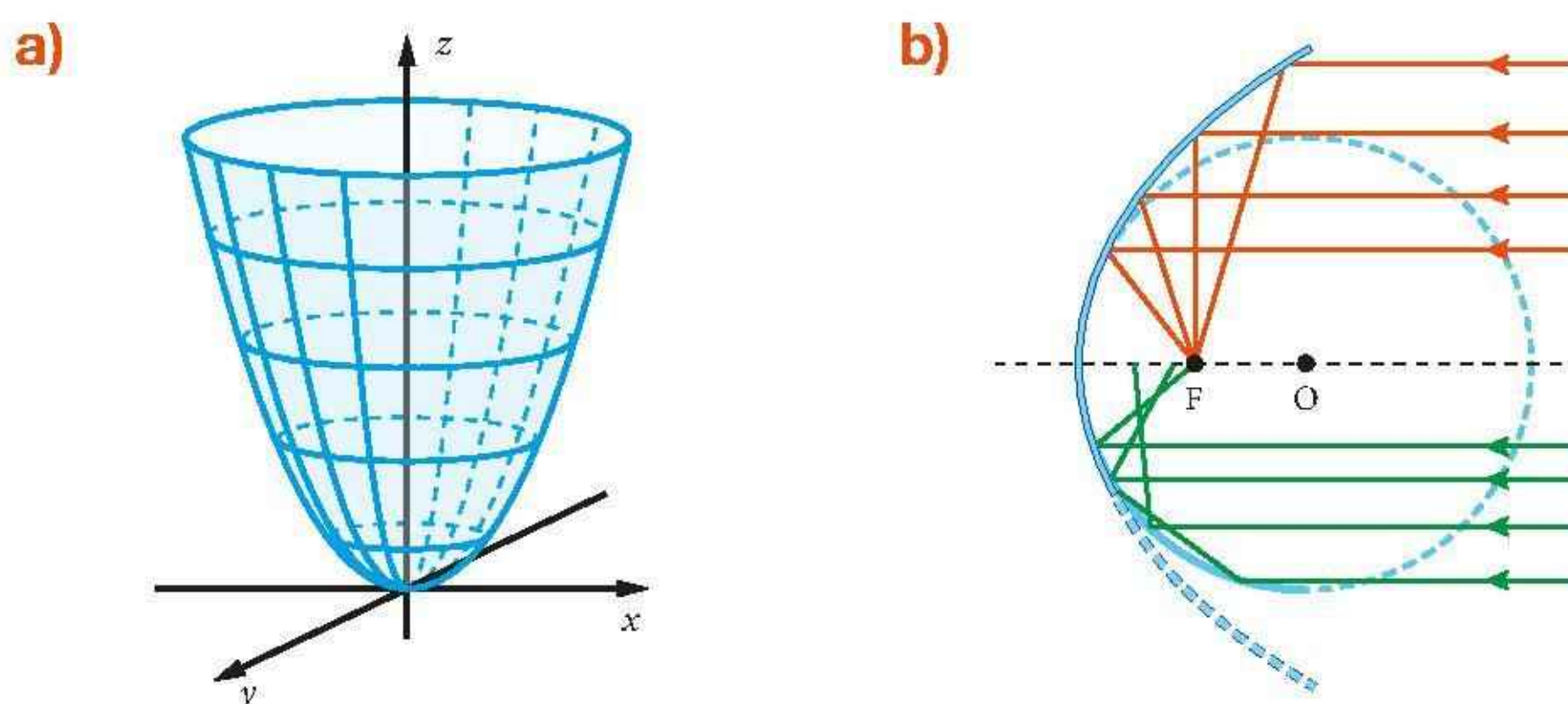
Rys. 16.82. Z zwierciadło paraboliczne: a) powstawanie paraboloidy, b) porównanie biegu promieni w zwierciadle sferycznym (kolor zielony) i parabolicznym (kolor czerwony)
