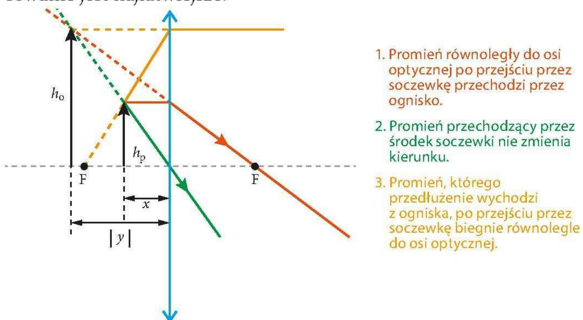
Rys. 16.74. Konstrukcja obrazu utworzonego przez soczewkę skupiającą, gdy przedmiot znajduje się bliżej soczewki, niż wynosi jej ogniskowa
