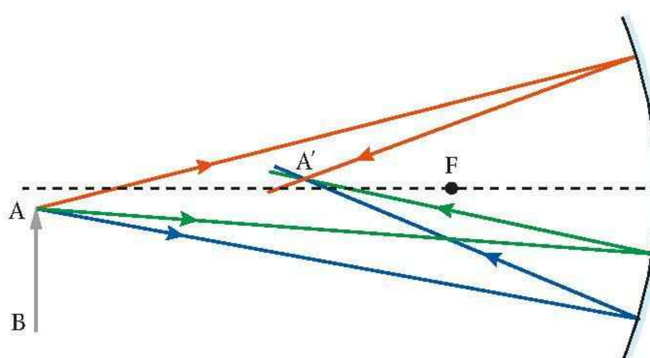
Rys. 16.83. Mechanizm tworzenia obrazu rzeczywistego przez zwierciadło wklęsłe
