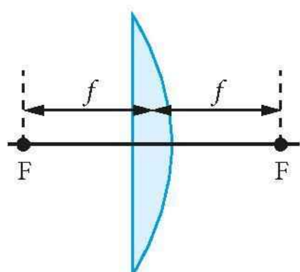
Rys. 16.62. Nawet w soczewce niesymetrycznej ogniska są położone w takich samych odległościach po obu stronach soczewki
