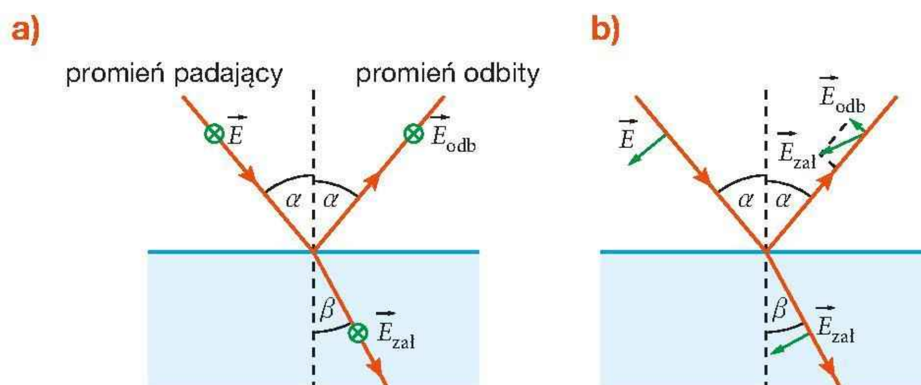
Rys. 16.108. Polaryzacja przez odbicie: a) promień padający spolaryzowany prostopadłe do płaszczyzny padania (czyli do płaszczyzny rysunku), b) promień padający spolaryzowany równoległy do tej płaszczyzny
