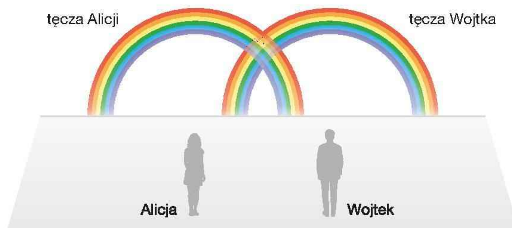
Rys. 16.55. Każdy obserwator widzi własną tęczę, powstającą w innych kropelkach wody
