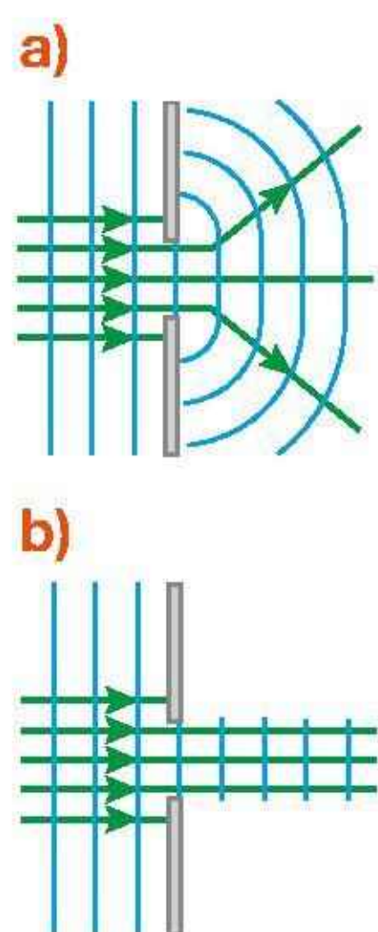
Rys. 16.15. Przejście światła przez otwór: a) z uwzględnieniem dyfrakcji (optyka falowa), b) w przybliżeniu w optyce geometrycznej
