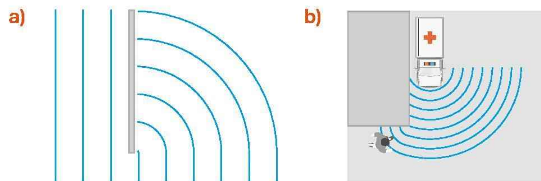
Rys. 16.12. Dyfrakcja fal mechanicznych: a) fale na wodzie, b) fale dźwiękowe (widok z góry)
