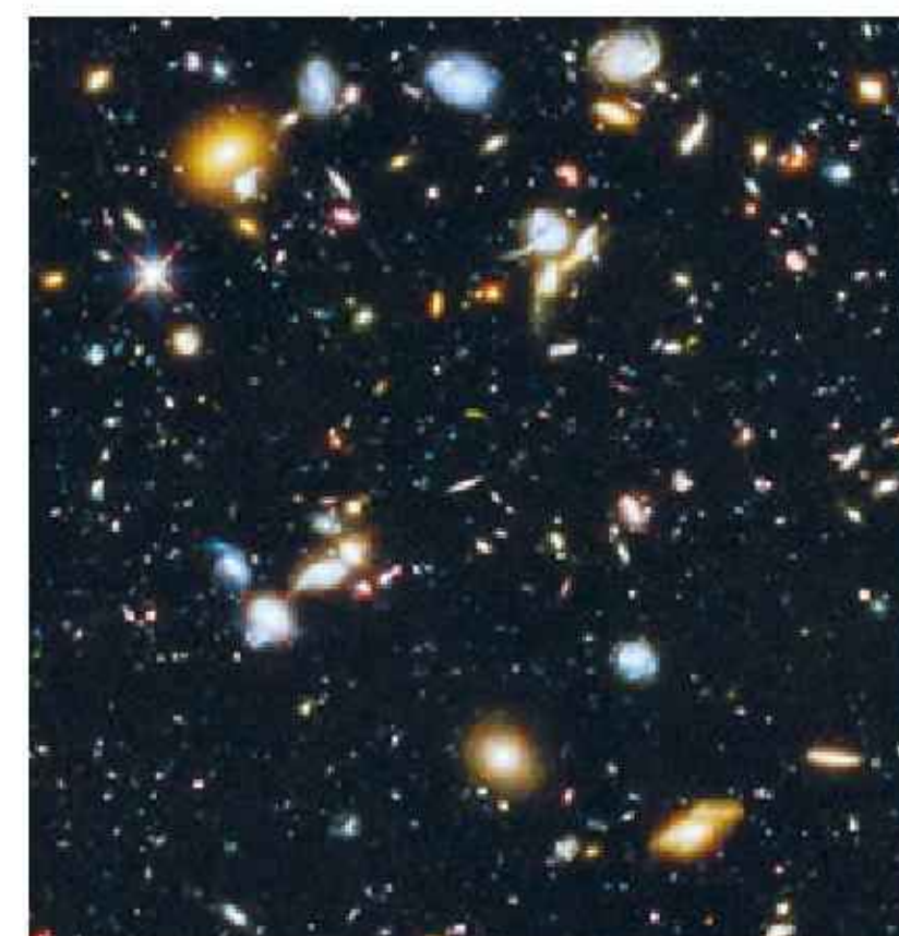
Rys. 18.38. Głębokie Pole Hubble'a, czyli zdjęcie niewielkiego obszaru z pozoru pustego nieba, które po naświetlaniu przez 10 dni ukazało bogactwo odległych, słabo widocznych galaktyk
