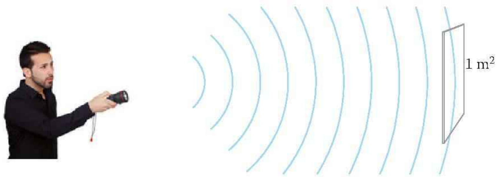
Rys. 16.4. Natężenie fali to energia fali padającej na 1 \text{ m}^2 w ciągu sekundy
