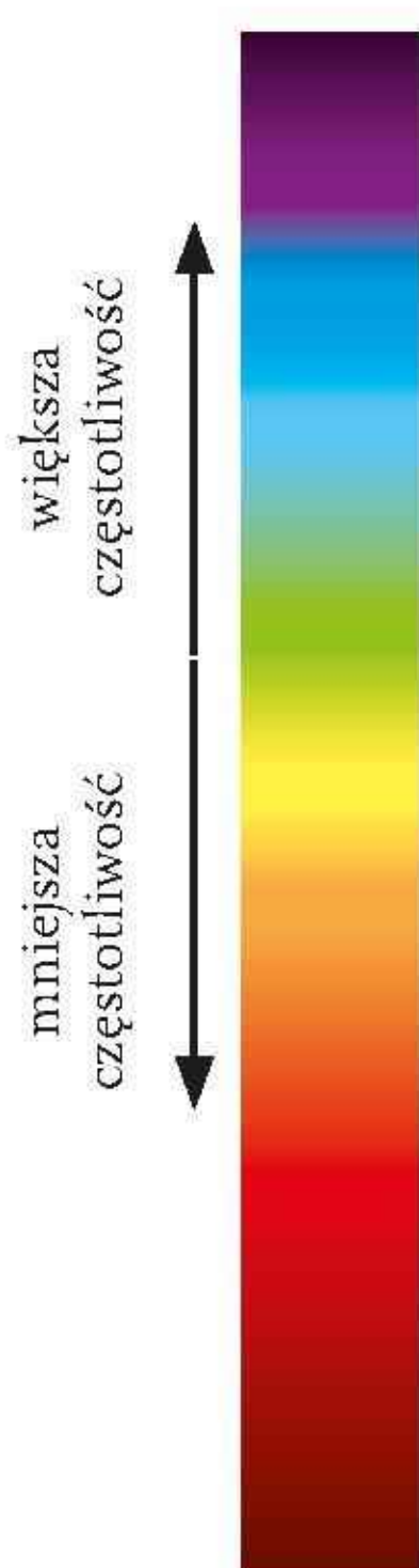
Rys. 19.24. Widmo światła białego i zmiana koloru zielonego w zależności od kierunku ruchu obiektu (oddala się lub zbliża)
