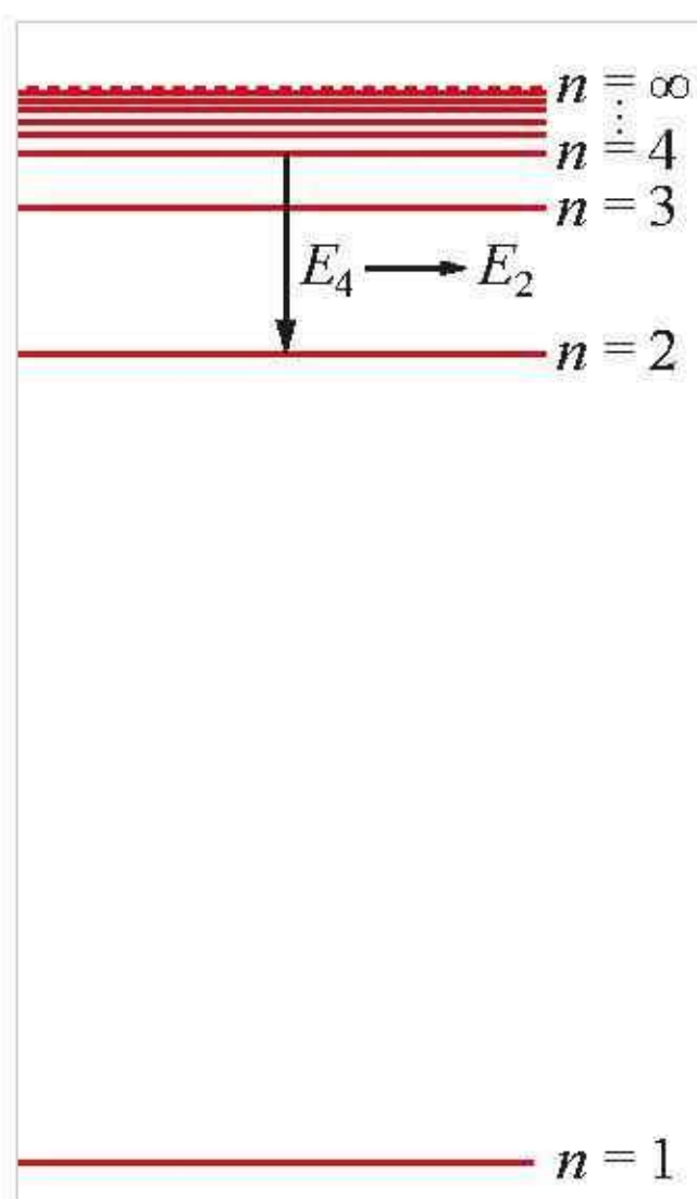
Rys. 17.37. Dozwolone energie atomu wodoru
