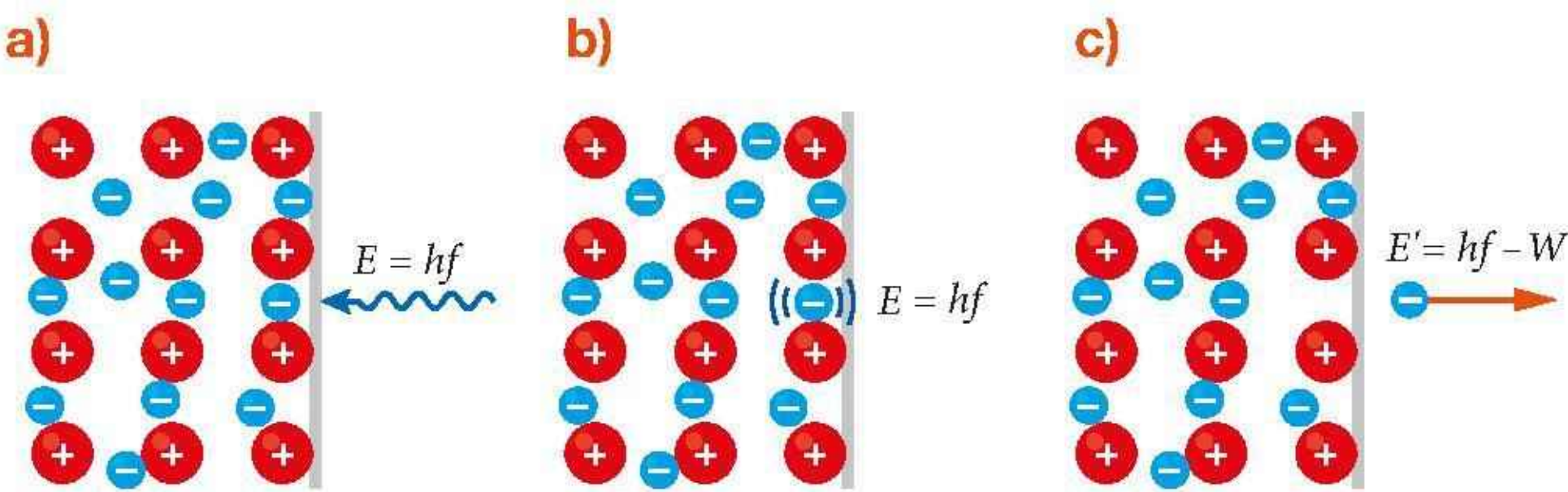
Rys. 17.21. Bilans energetyczny zjawiska fotoelektrycznego: a) foton o energii hf pada na powierzchnię metalu, b) elektron pochłania energię fotonu, c) wybity elektron ma energię kinetyczną mniejszą o W od energii fotonu
