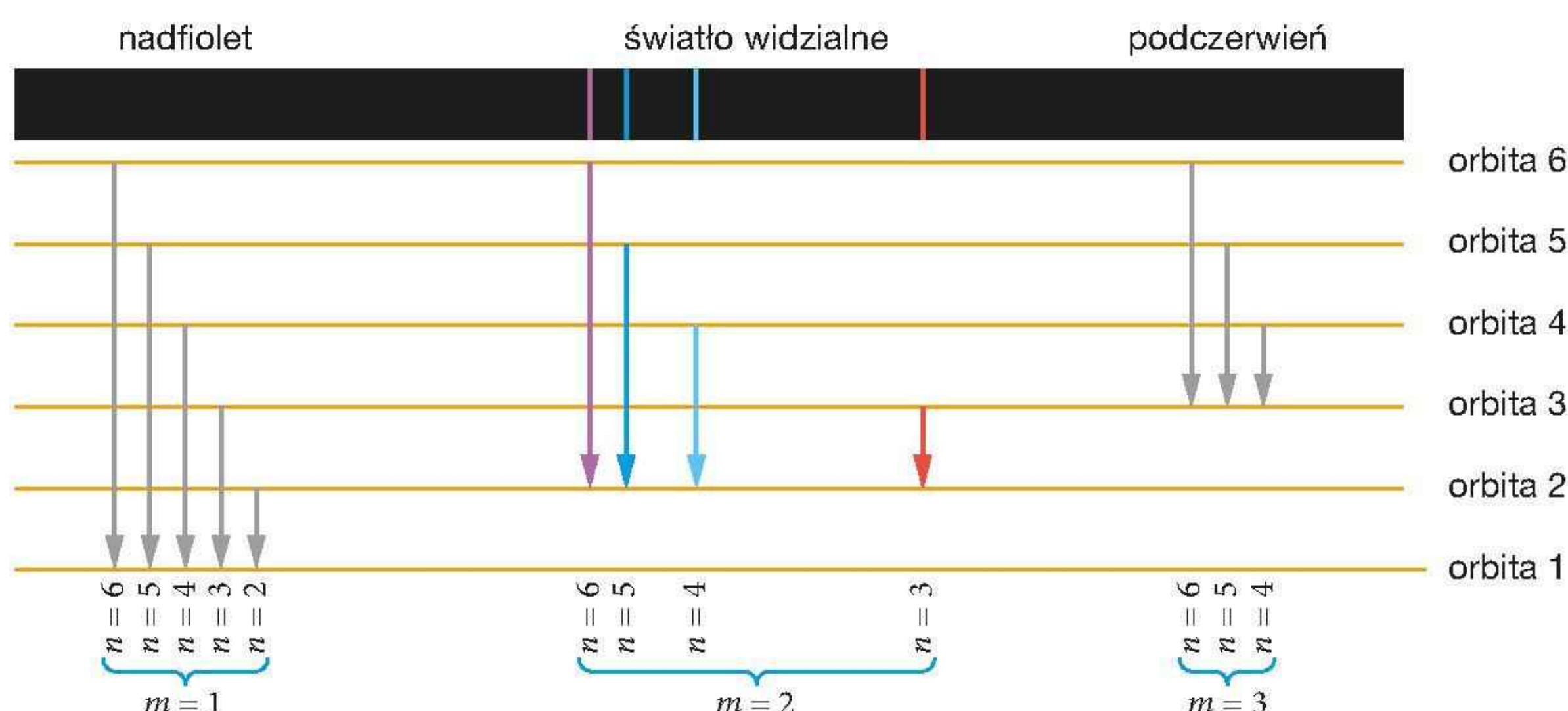
Rys. 17.33. Widmo atomu wodoru składa się z prążków o określonych długościach fali (odległości między orbitami nie zachowują skali)
