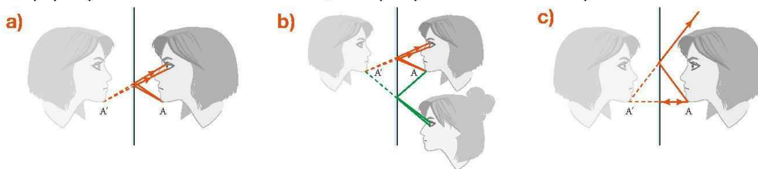
Rys. 16.77. Obraz pozorny w zwierciadle: a) mechanizm powstawania, b) niezależność położenia obrazu od położenia obserwatora, c) najprostsza konstrukcja
