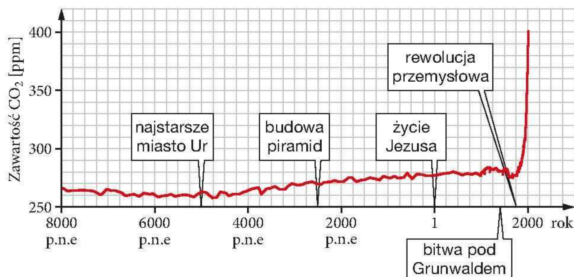
Rys. 17.15. Koncentracja \text{CO}_2 w atmosferze wyrażona w częściach milionowych (ppm – parts per milion)
