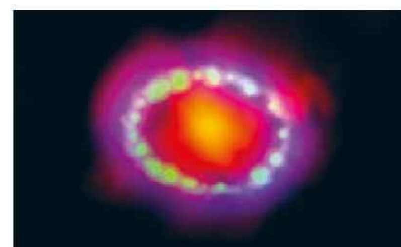
Rys. 18.36. Ostatnia supernowa (do 2021 r.) była widoczna z Ziemi gołym okiem w 1987 r. Zdjęcie pozostałości po wybuchu (2017 r.)
