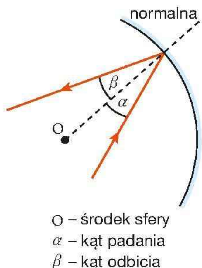
Rys. 16.78. Odbicie promienia światła od zwierciadła wklęsłego
