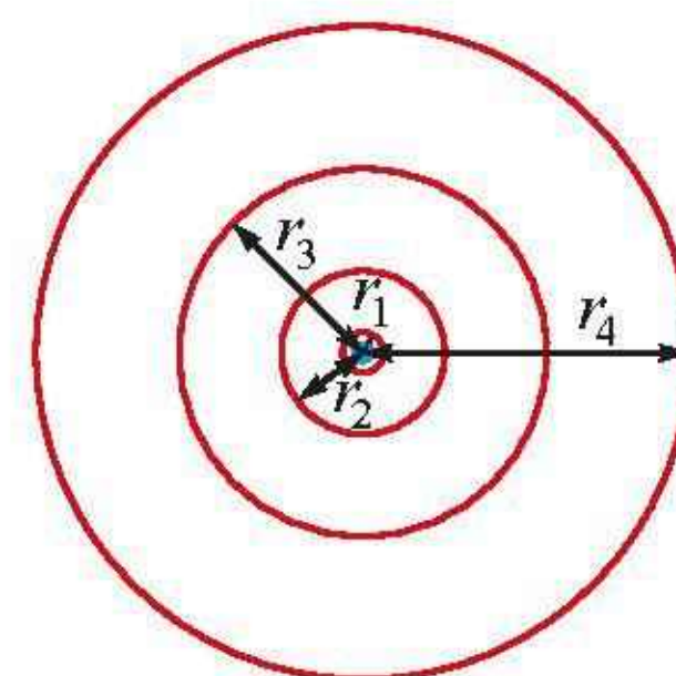
Rys. 17.36. Pierwsze cztery spośród dozwolonych orbit elektronowych w atomie wodoru
