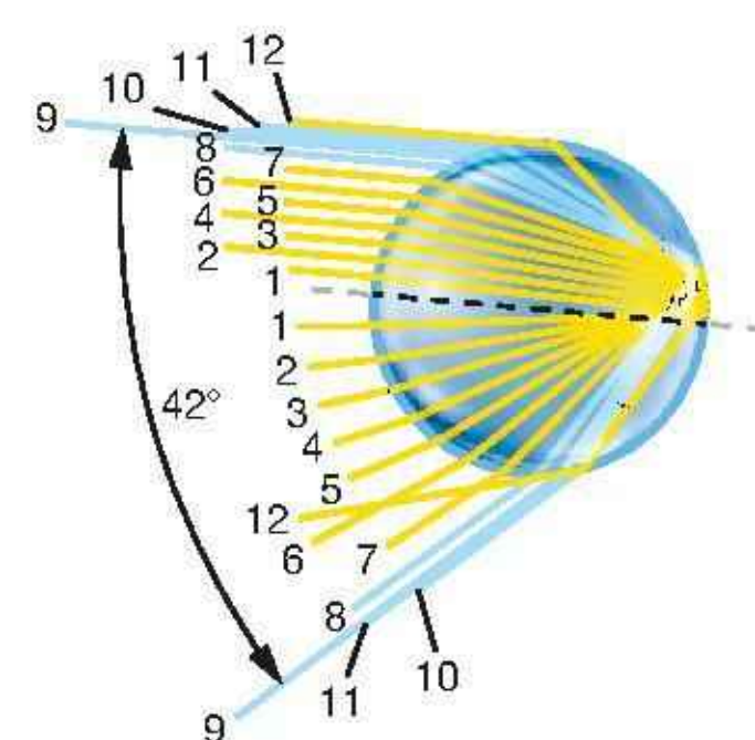
Rys. 16.53. Załamanie poszczególnych promieni w kropli wody w zależności od miejsca padania promieni
