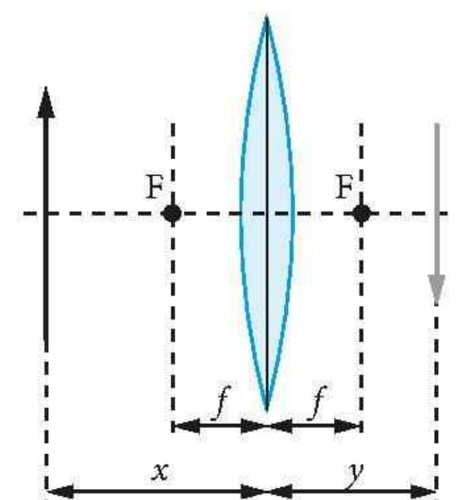
Rys. 16.69. Ogniskowa soczewki ( f ), odległość przedmiotu od soczewki ( x ), odległość obrazu od soczewki ( y )
