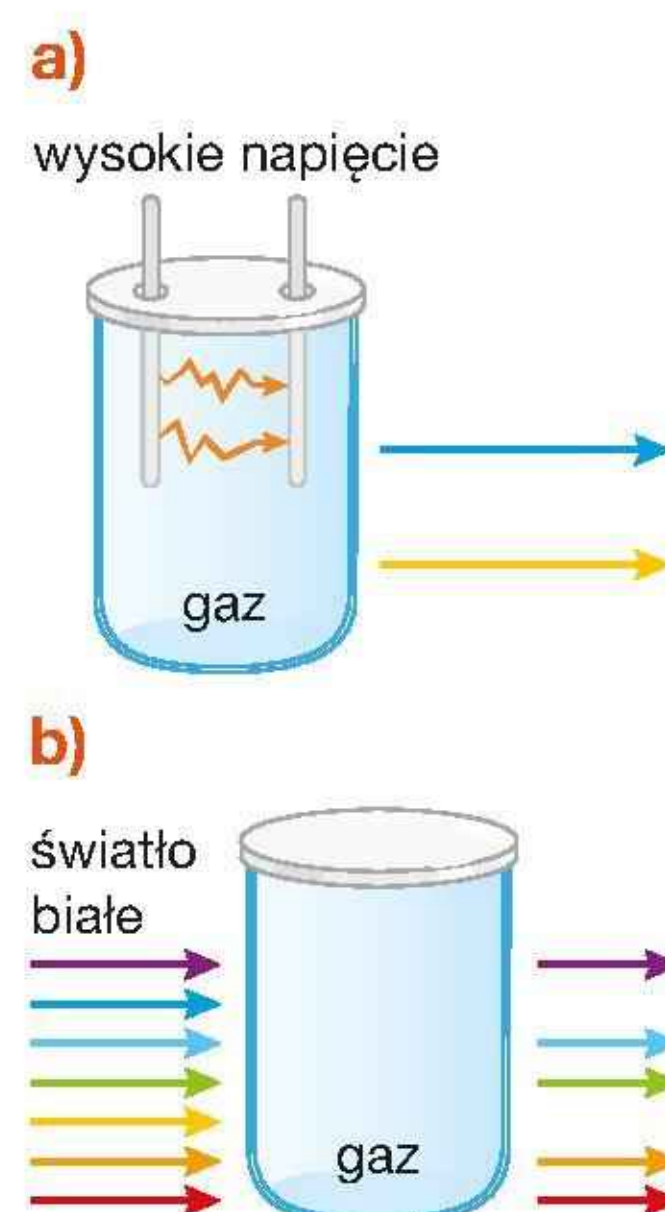
Rys. 17.29. Powstawanie widma: a) emisyjnego, b) absorpcyjnego
