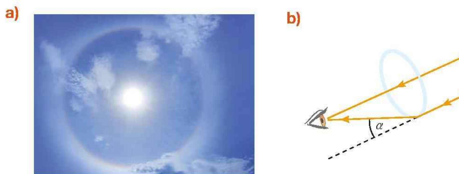
Rys. 16.56. Halo słoneczne (a) i schemat jego powstawania (b)
