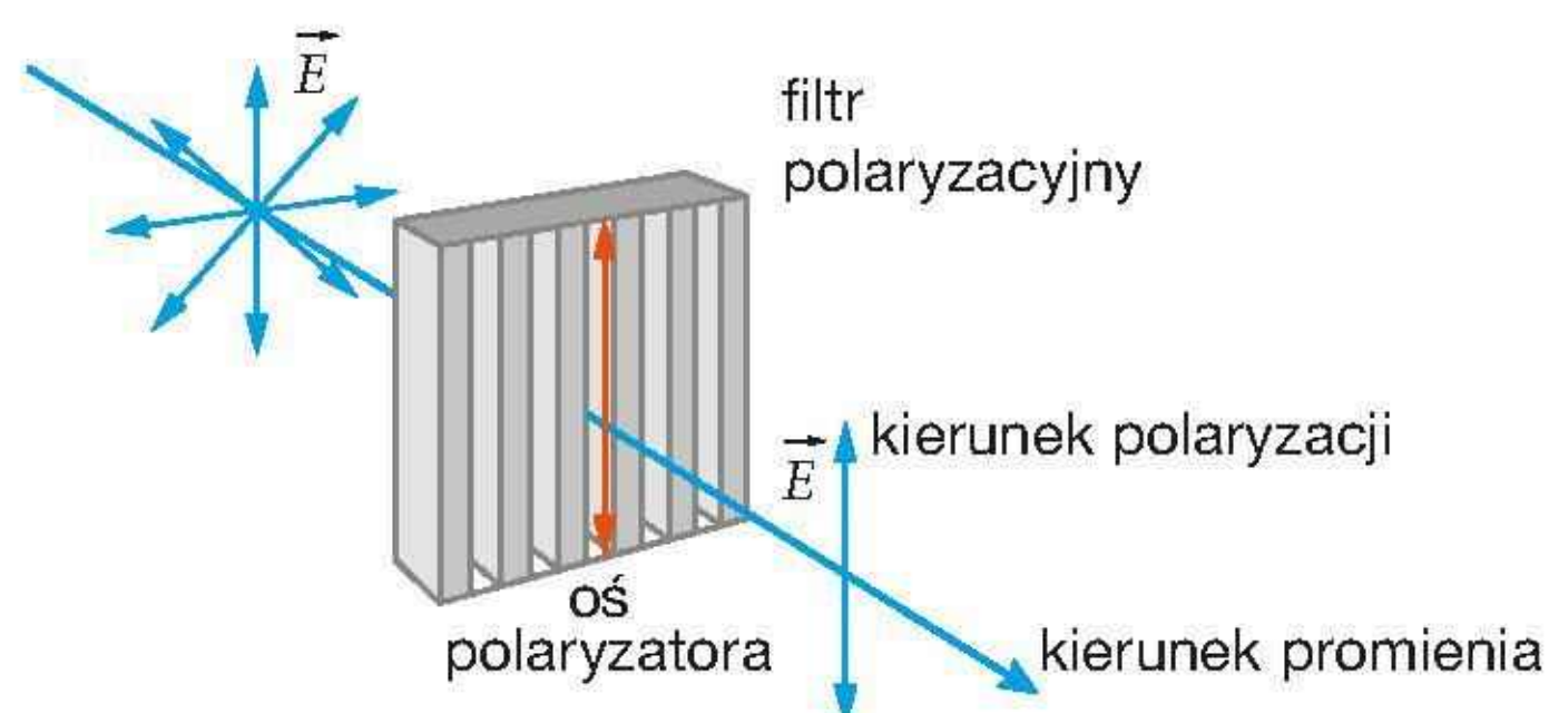
Rys. 16.103. Schemat działania filtra polaryzacyjnego
