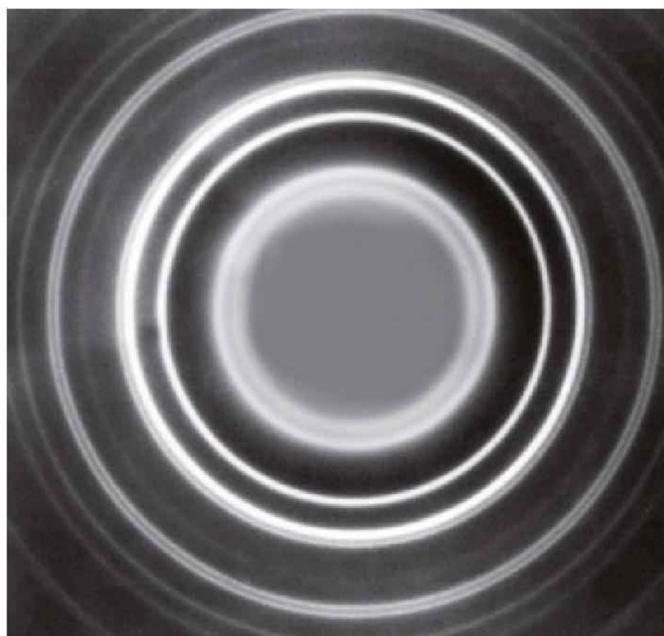
Rys. 17.25. Obrazy interferencyjne uzyskane po dyfrakcji elektronów na sieci krystalicznej cyrkonu (a) i promieniowania rentgenowskiego na kryształach złota (b). Białe i czarne obszary odpowiadają wzmacnianiu i wygaszaniu się fali
