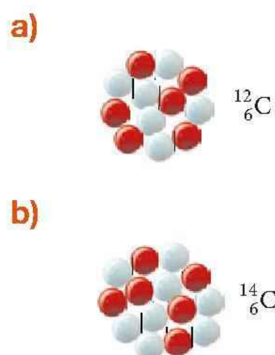
Rys. 18.2. Schematyczny rysunek jądra węgla (protony – czerwone): a) ^{12}_6\text{C} , b) ^{14}_6\text{C}
