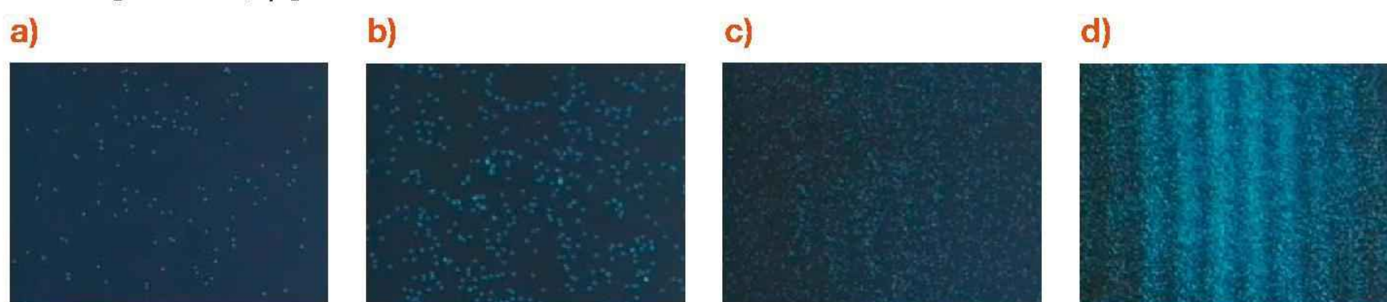
Rys. 17.26. Tworzenie obrazu interferencyjnego przez elektrony
