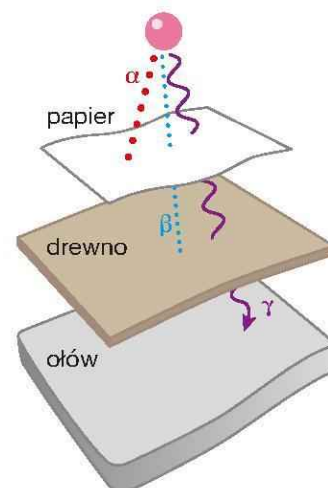
Rys. 18.4. Przenikliwość poszczególnych rodzajów promieniowania
