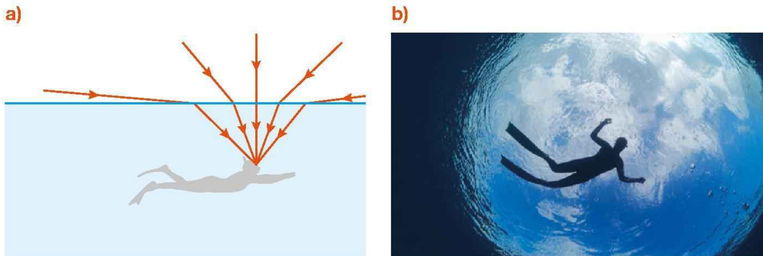
Rys. 16.49. Okno Snelliusa: a) mechanizm powstawania, b) zdjęcie spod wody
