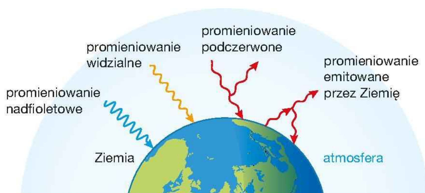
Rys. 17.14. Powstawanie efektu cieplarnianego
