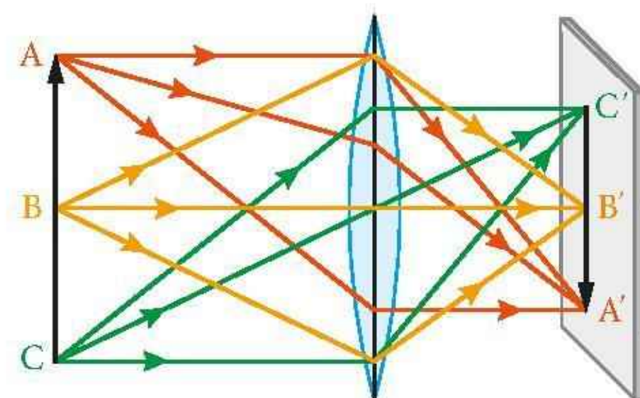
Rys. 16.66. Tworzenie obrazu rzeczywistego przez soczewkę skupiającą: a) układ doświadczalny, b) schemat wyjaśniający przebieg zjawiska
