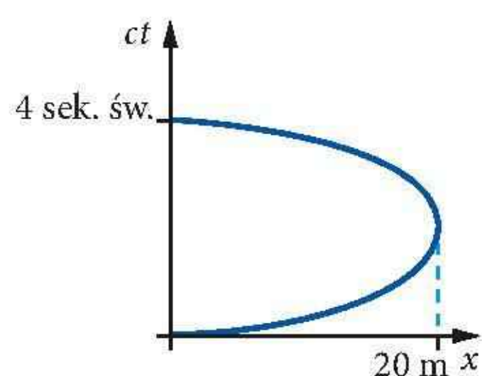
Rys. 19.26. Trajektoria piłeczki rzuconej do góry
