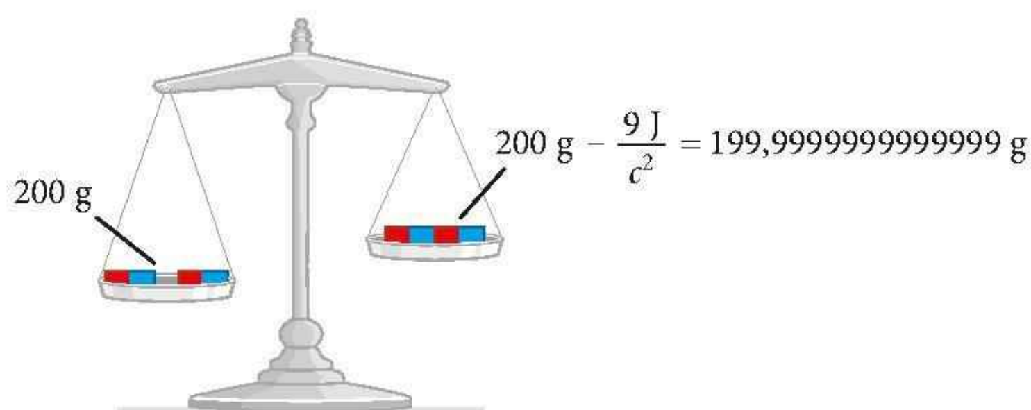
Rys. 18.23. Jeśli przy rozłączaniu magnesów wykonujemy pracę 9 J, to masa złączonych magnesów jest o 9 \frac{J}{c^2} = 10^{-13} \text{ g} mniejsza niż rozłączonych
