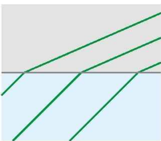
Rys. 16.37. Na granicy ośrodków grzbiety fal tworzą linie ciągłe
