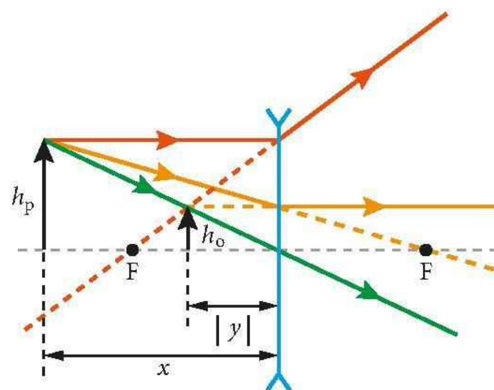
Rys. 16.76. Konstrukcja obrazu tworzonego przez soczewkę rozpraszającą
