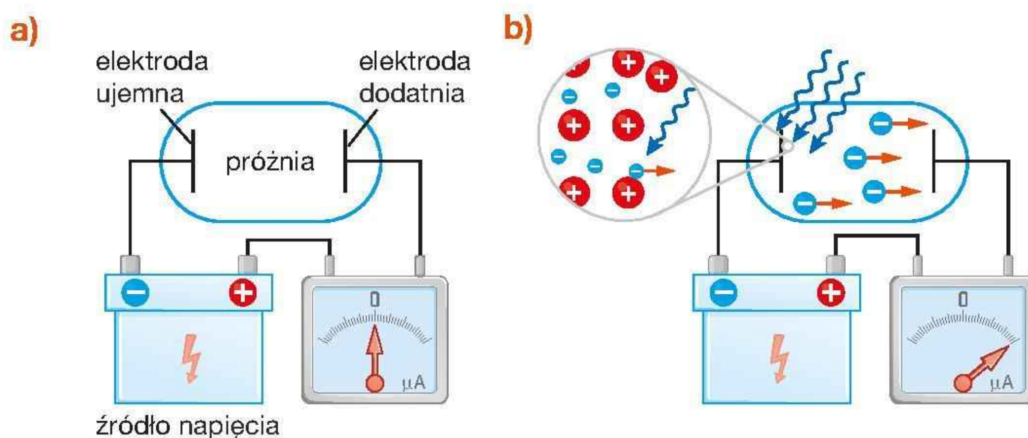
Rys. 17.18. Układ do badania zjawiska fotoelektrycznego
