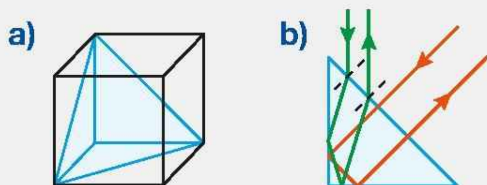
Rys. 3. Reflektor rogowy (a), odbicie współdrożne w reflektorze rogowym (b)
