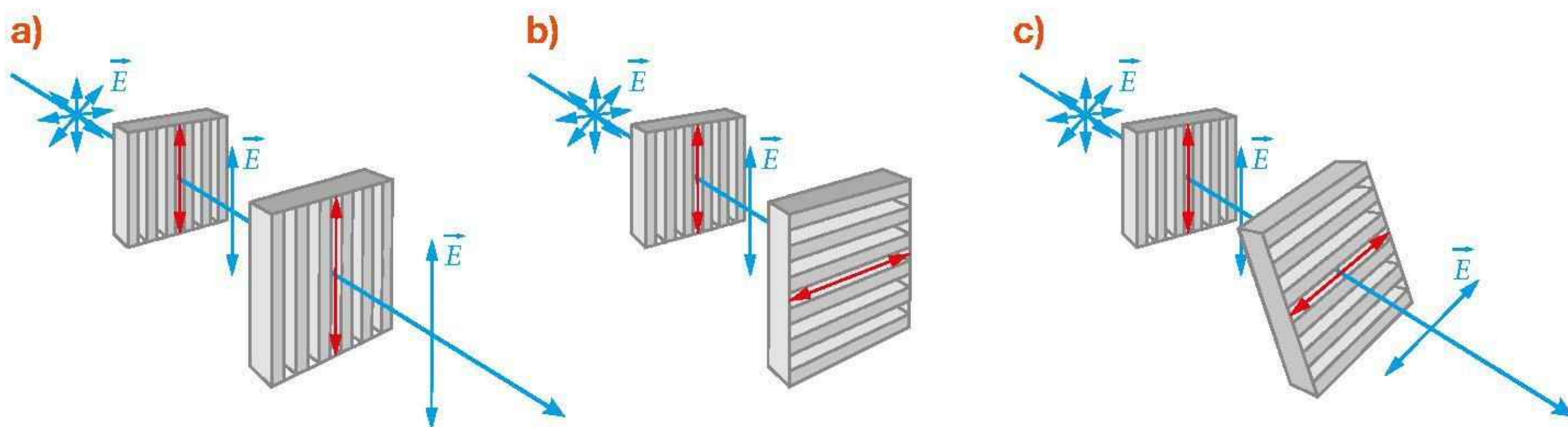
Rys. 16.104. Przejście światła przez dwa kolejne filtry polaryzacyjne
