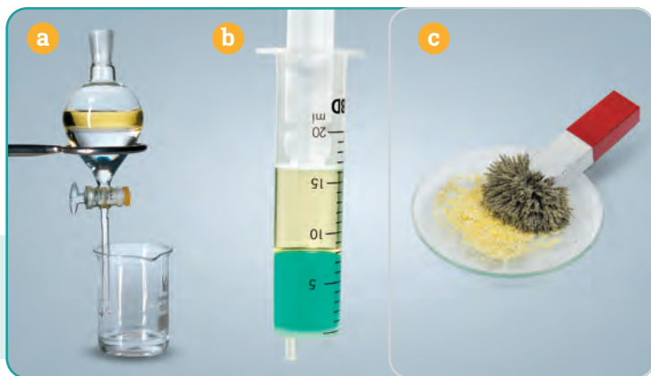
Rozdzielanie rozdzielaczem (a), strzykawką (b) i magnesem (c)
