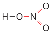
kwas azotowy(V)
