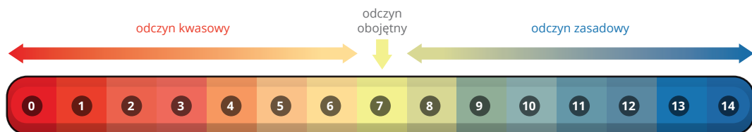
Skala pH z barwami wskaźnika uniwersalnego
