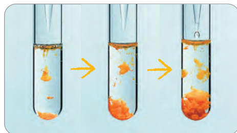
Strącanie się osadu siarczku kadmu
