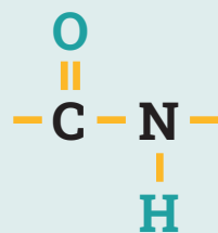
Wiązanie peptydowe
