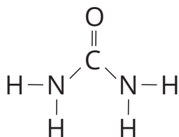
Wzór mocznika
