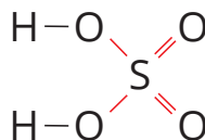
kwas siarkowy(VI)
