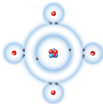
Model cząsteczki metanu
