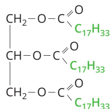
trioleinian glicerolu
