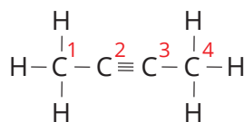
Wzór but-2-ynu
