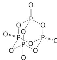
Wzór strukturalny tlenku fosforu(V)
