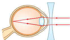
krótkowidz
