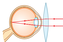
dalekowidz
