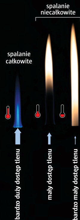
▲ Płomień palnika gazowego w warunkach różnego dostępu powietrza
