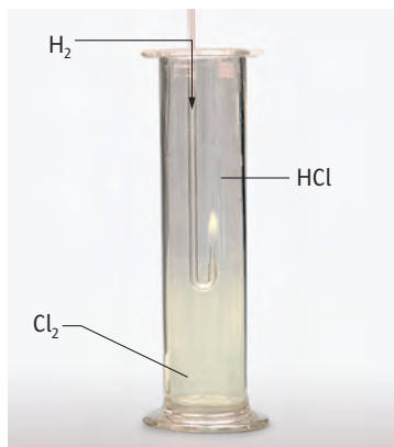
▲ Otrzymywanie chlorowodoru – reakcja spalania wodoru w chlorze
