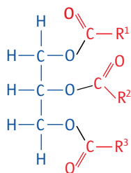
wzór ogólny strukturalny tłuszczów
