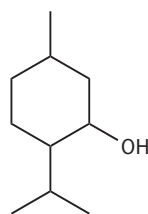
mentol
