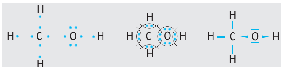
▲ Schemat tworzenia wiązań chemicznych w cząsteczce metanolu
