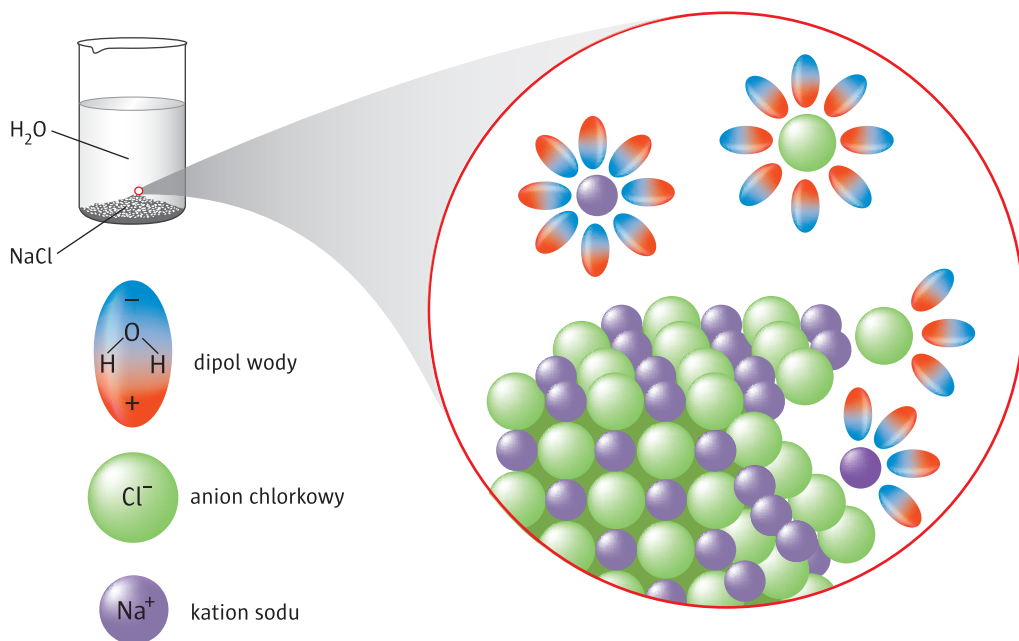
▲ Dysocjacja elektrolityczna chlorku sodu
