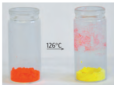
▲ Jodek rtęci(II)
