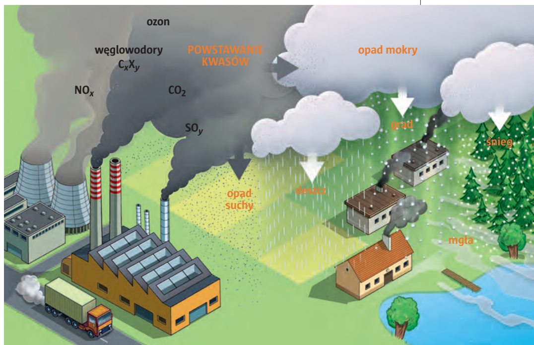
▲ Powstawanie kwaśnych opadów
