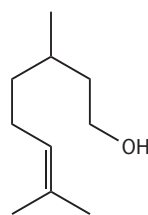
cytronelol
