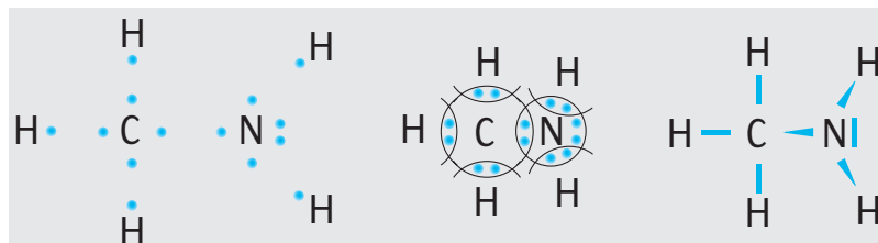
▲ Schemat tworzenia wiązań chemicznych w cząsteczce metyloaminy
