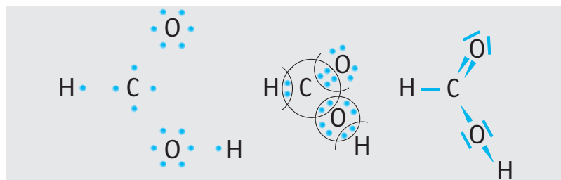
▲ Schemat tworzenia wiązań chemicznych w cząsteczce kwasu metanowego
