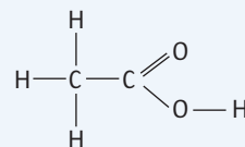
wzór strukturalny
