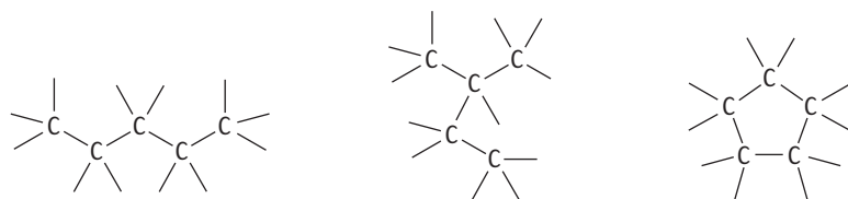
łańcuch nierozgałęziony
