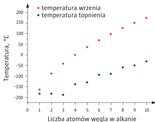
◀ Wykresy przedstawiające zmiany temperatury wrzenia i temperatury topnienia w szeregu homologicznym alkanów
