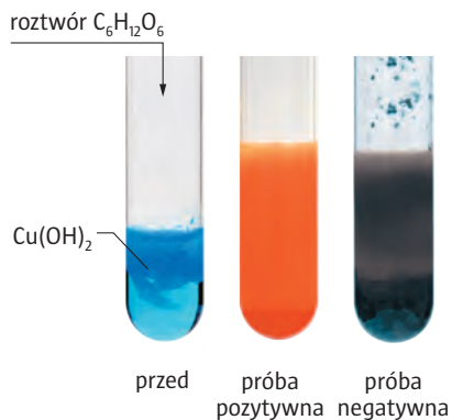
▲ Reakcja charakterystyczna glukozy
