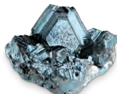
Sfaleryt, \text{ZnS}
