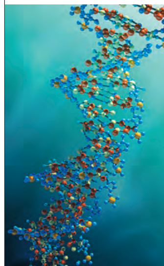
▲ Struktura DNA
