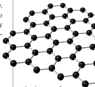
▲ Struktura grafenu, który jest postacią pierwiastkową węgla
