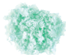
FeSO 4
