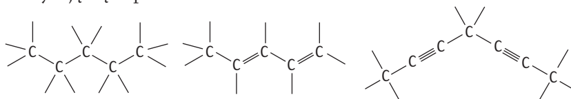
wiązania pojedyncze
