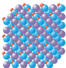
▲ Sieć krystaliczna NaOH
