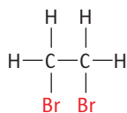
1,2-dibromoetan
