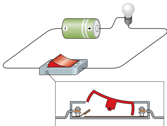
Prąd nie popłynie
