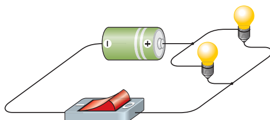
Połączenie równoległe
