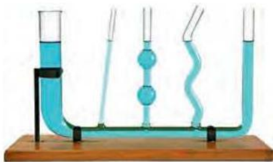
Przykład naczyń połączonych.
