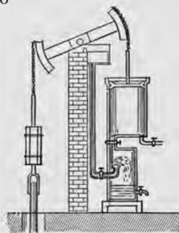
Silnik parowy Jamesa Watta.
