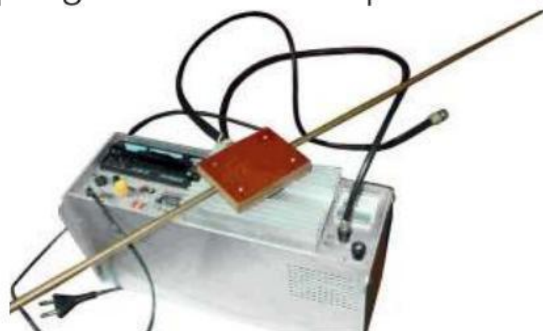
Przenośny nadajnik radiowy Berta.
