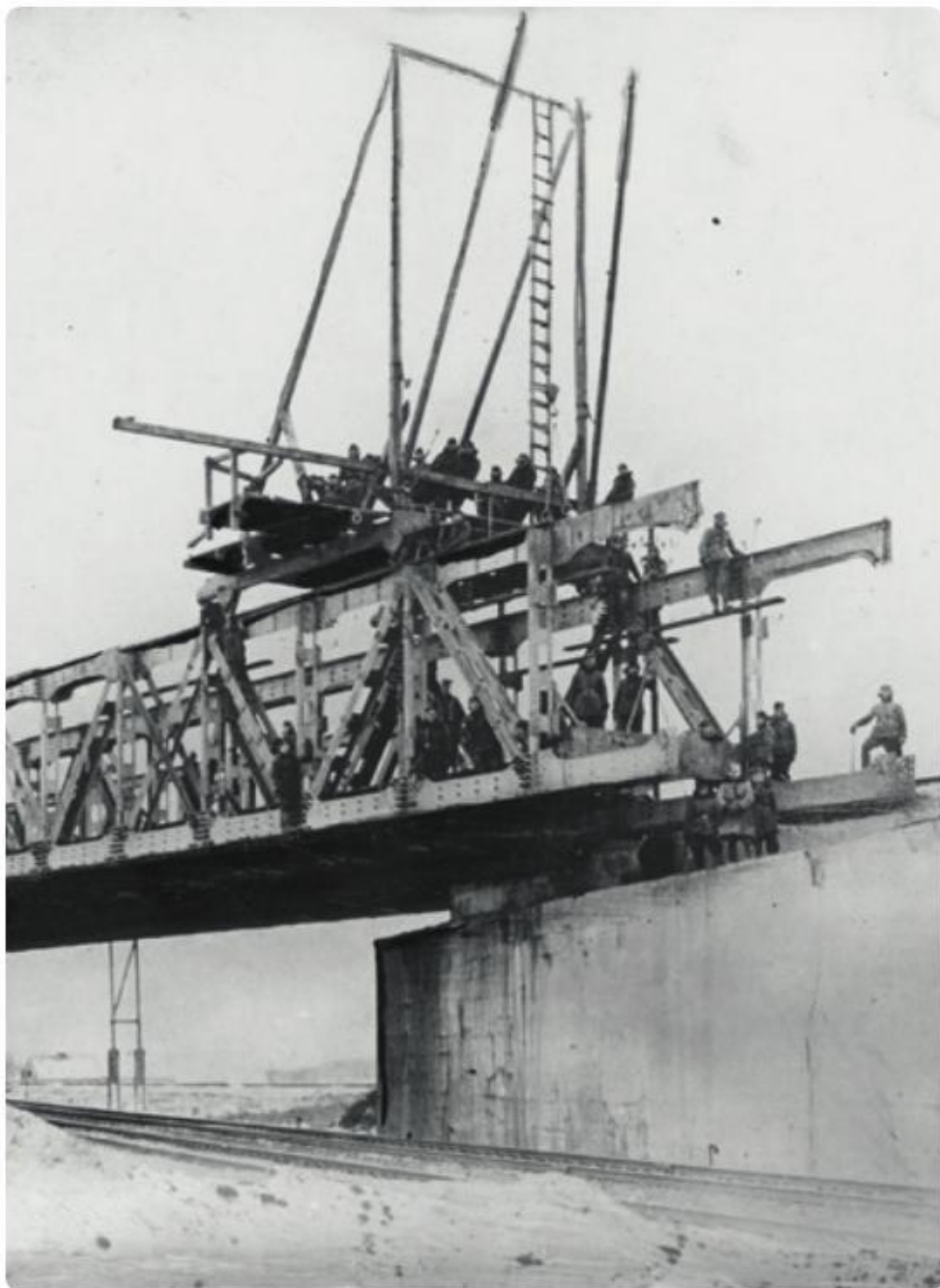
Budowa wiaduktu w Tczewie (Pomorze) dla magistrali węglowej łączącej Śląsk z Gdynią. Zdjęcie z 1928 r.
